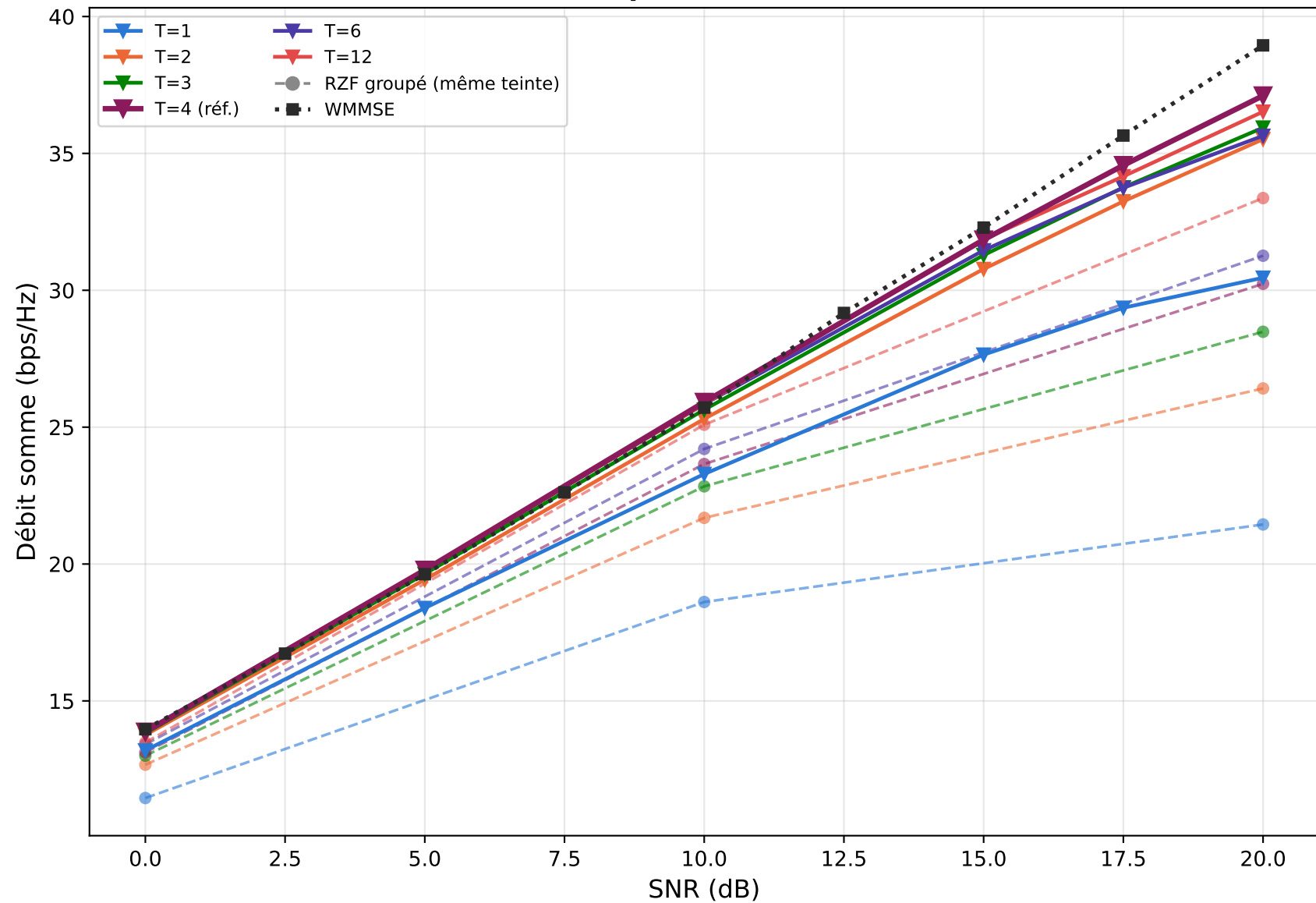
Débit somme vs SNR par T — TA-RB, UMi (M=8, K=4)
