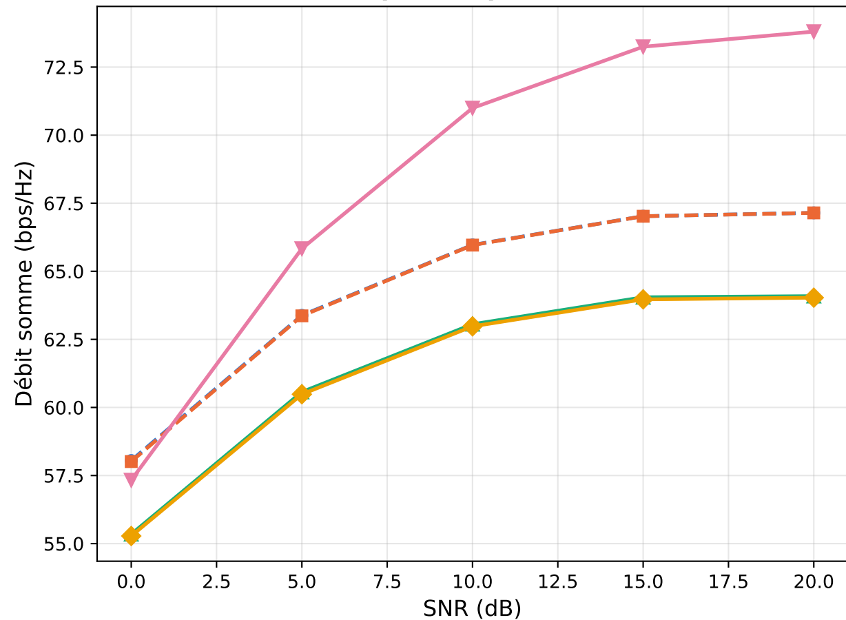
CSI imparfait (pilote 20dB)
