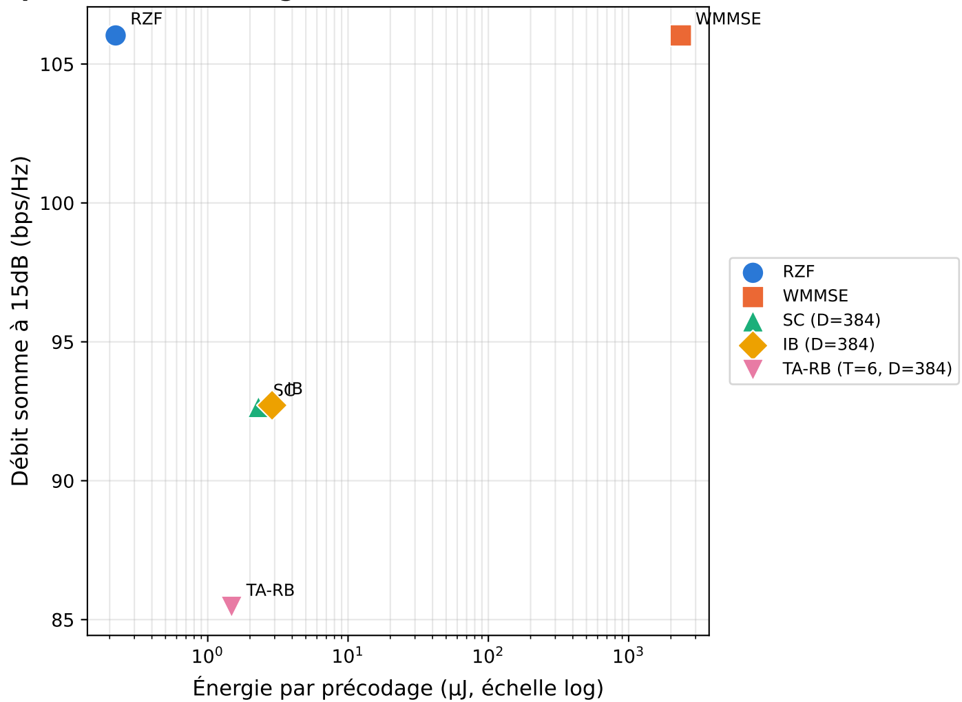
Compromis débit / énergie — UMa MASSIVE (M=64, K=8), D=384
