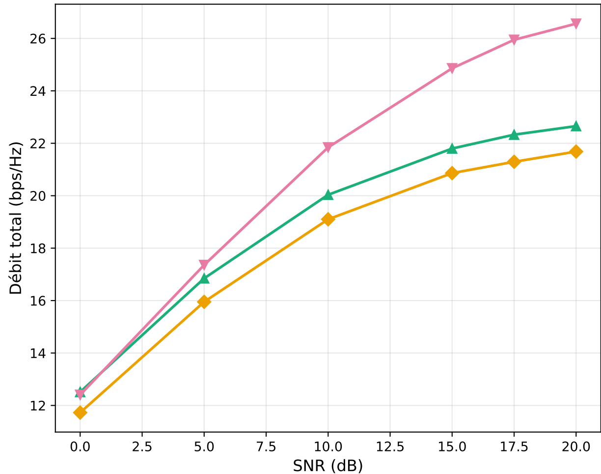
CSI imparfait (pilote 20dB) -- NON corrige
