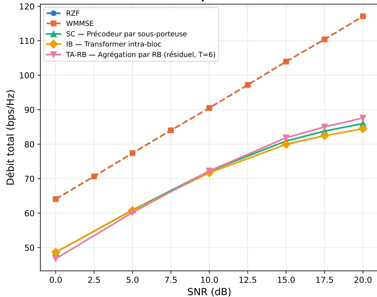
CSI parfait
