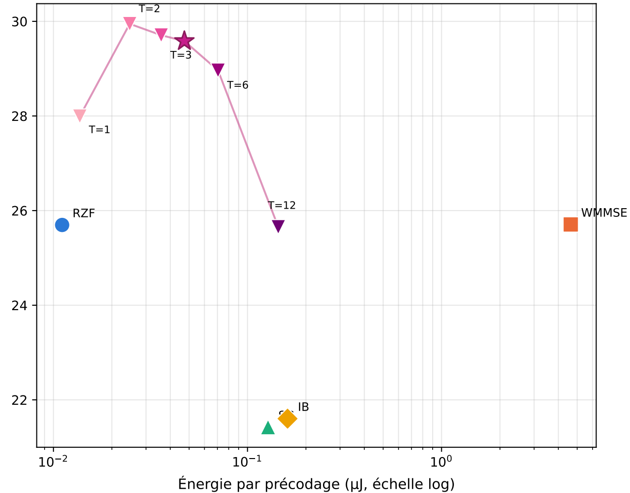
CSI imparfait (pilote 20dB)
