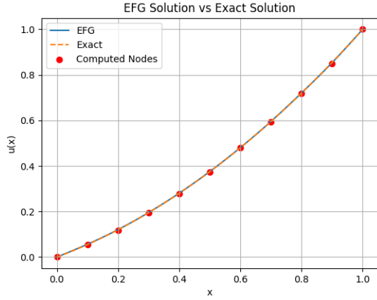
图 4.1 基于伽辽金型无网格方法的一维弹性杆问题数值结果
