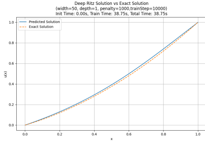
(a) 深度 Ritz 法-10000 步训练
