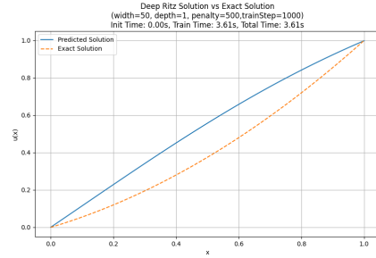
(b) 深度 Ritz 法-1000 步训练
