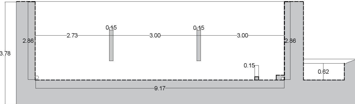
Longitudinal cut
