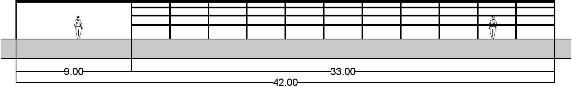
Longitudinal Section
