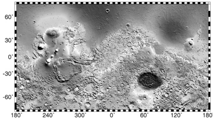
Figure 7-6: Latitude ( y -axis) and longitude ( x -axis) on Mars
