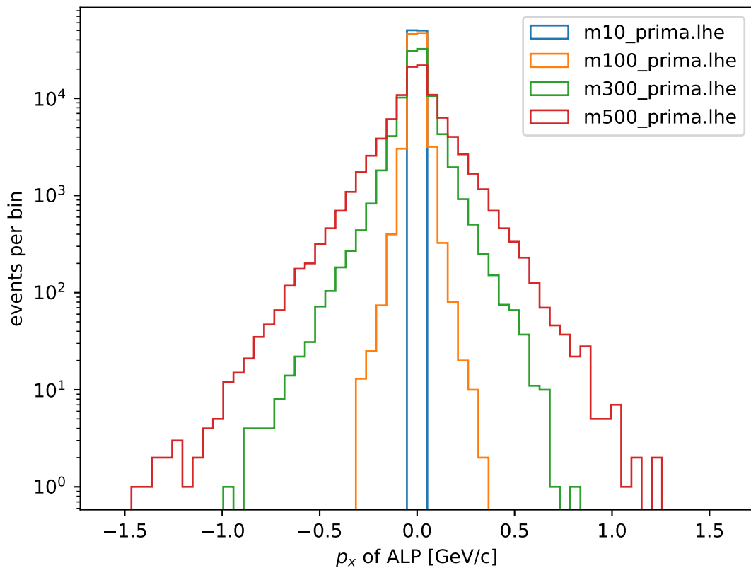
prima ALP p_x
