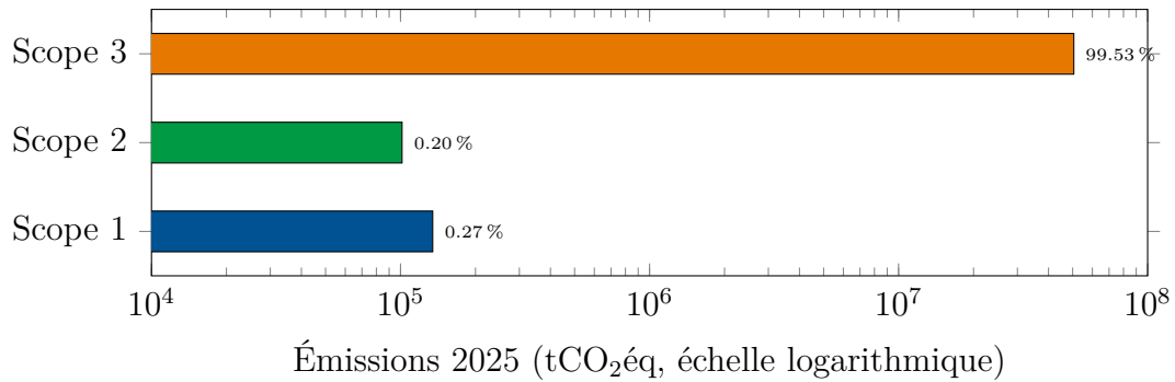
FIGURE 3 – Empreinte carbone d'Iveco Group en 2025 : répartition des émissions Scope 1, 2 et 3 en échelle logarithmique. Le Scope 3 domine avec 99,5 % du total, ce qui met en évidence la prédominance de la phase d'usage des véhicules vendus.
