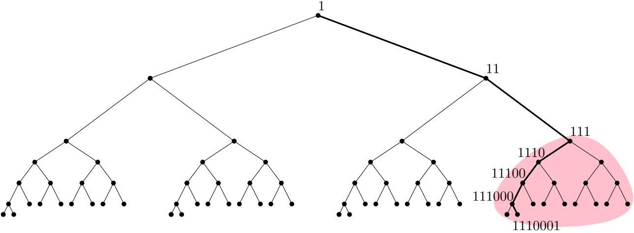
具有 2^2 \times (2^3 + 1) 的叶子的线段树
