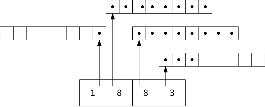
std::deque 的结构示意图
