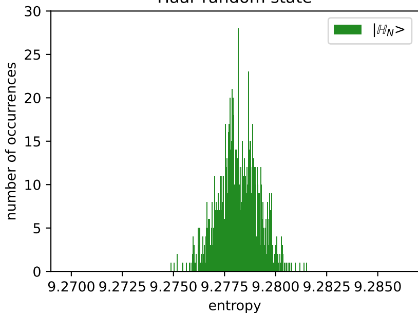
Haar random state
