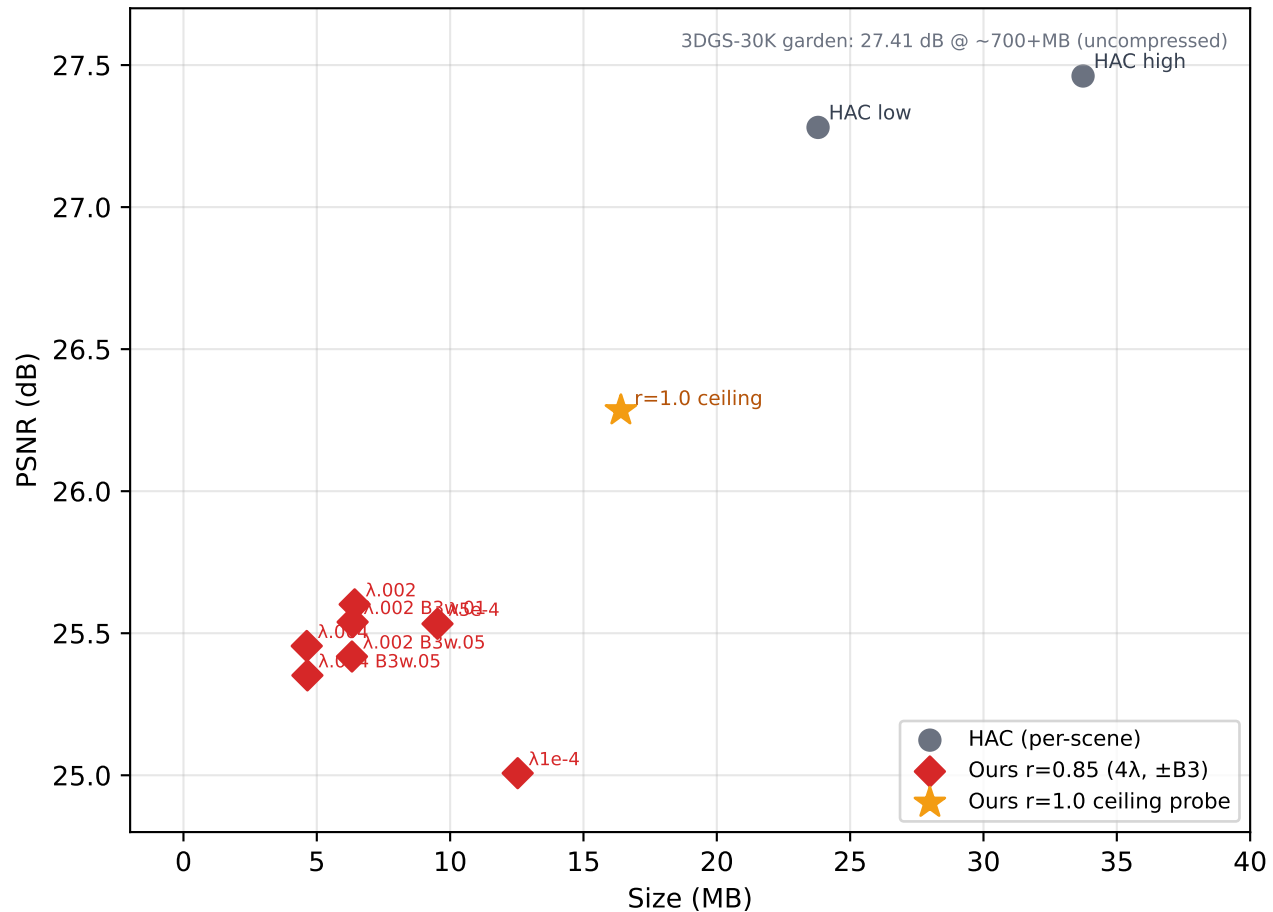
Mip-NeRF360: garden (r=2, 30k, seed 42)
