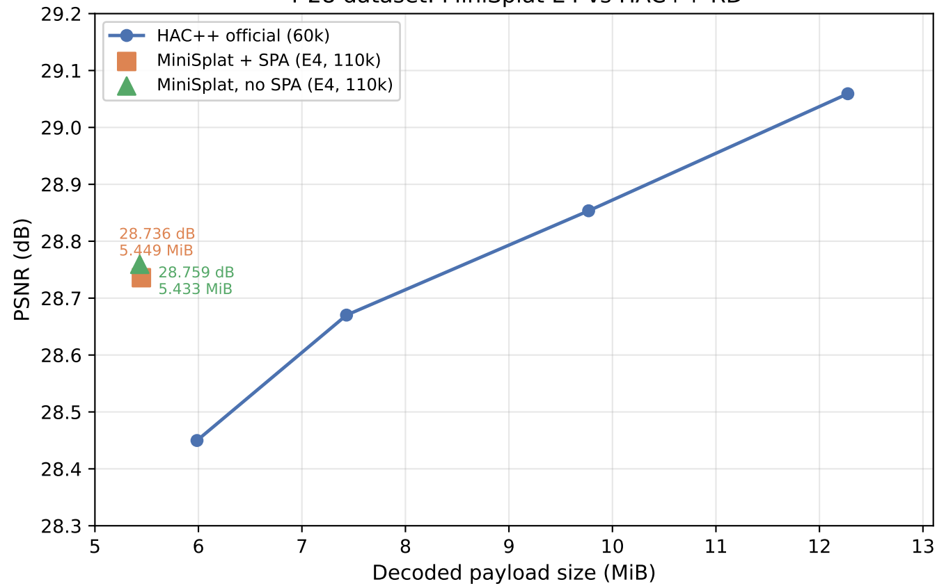
4-28 dataset: MiniSplat E4 vs HAC++ RD
