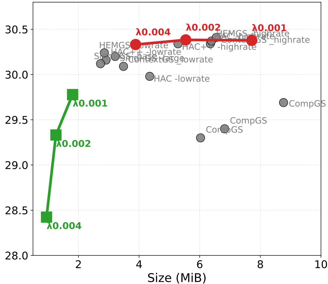
DB RD: PSNR vs Size
