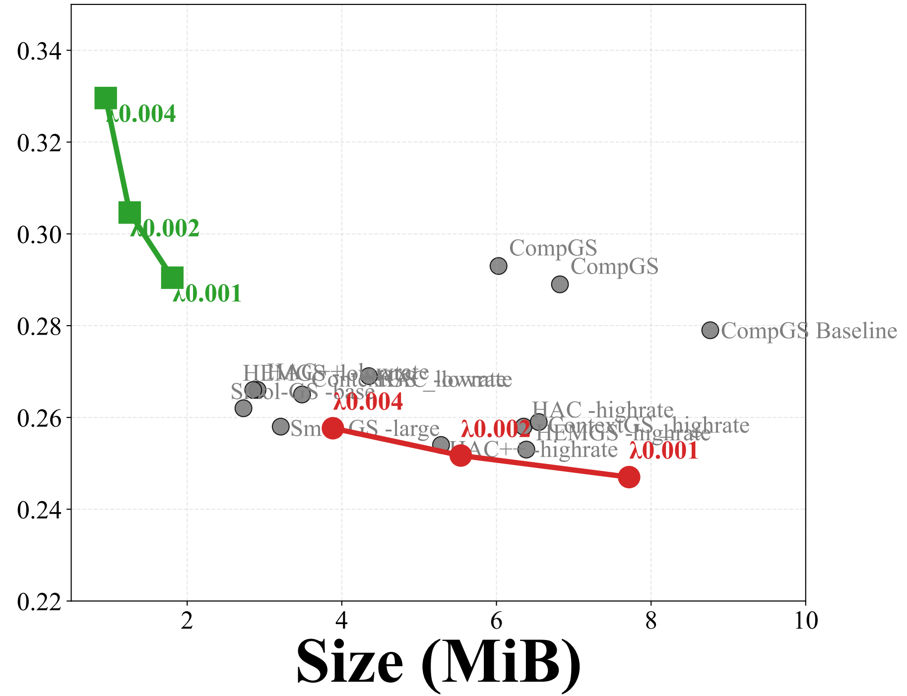
DB RD: LPIPS vs Size
