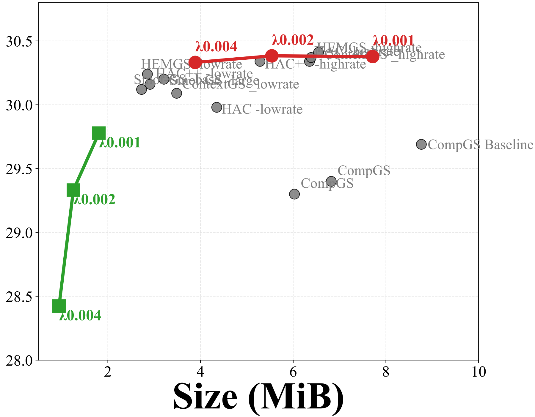
DB RD: PSNR vs Size
