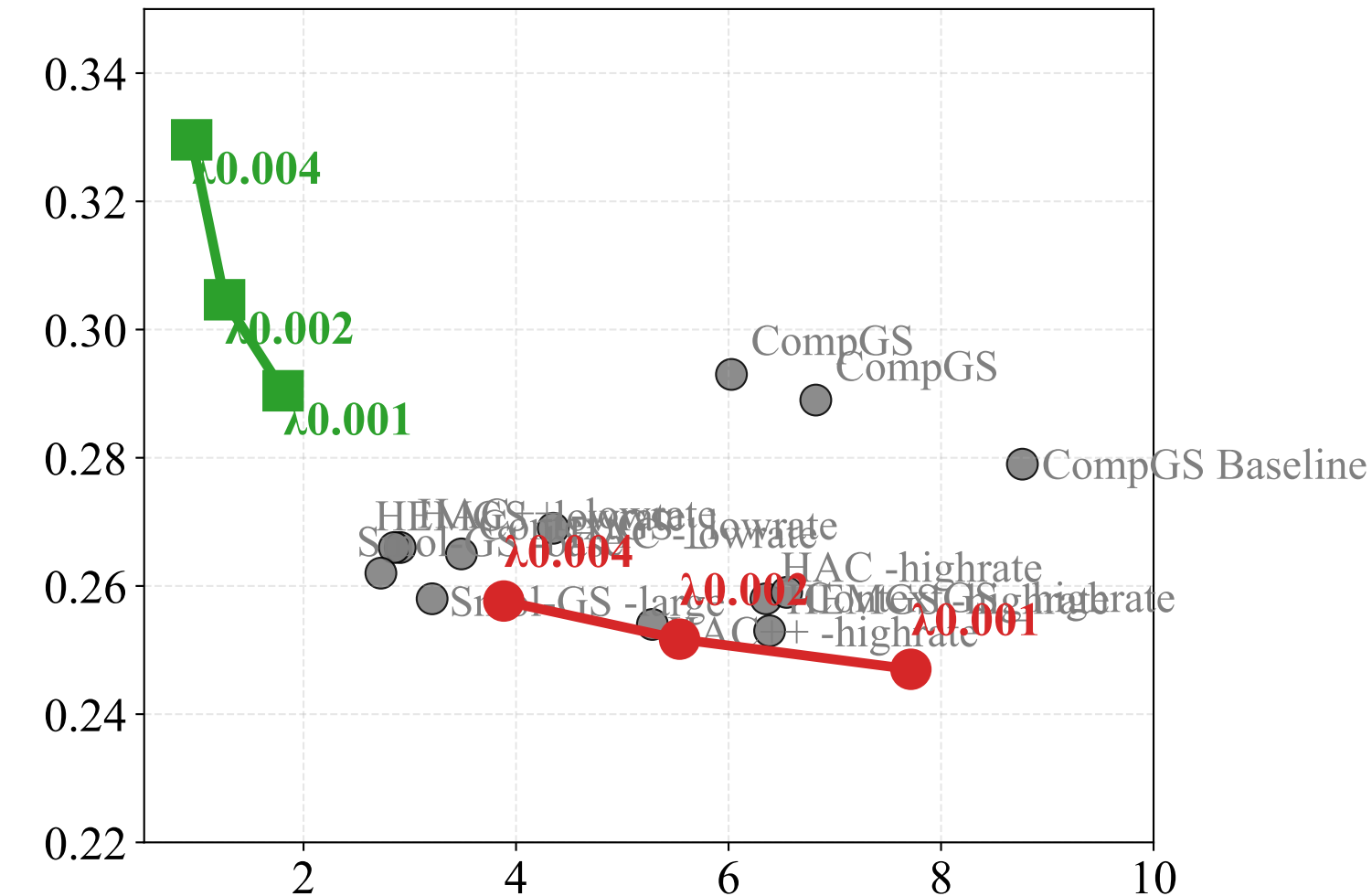
DB RD: LPIPS vs Size
