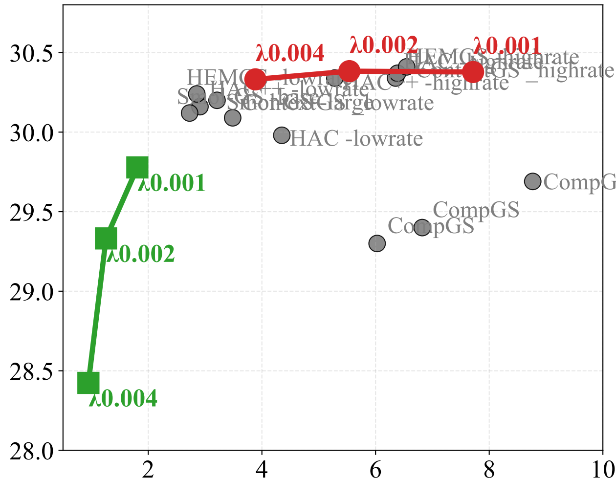
DB RD: PSNR vs Size
