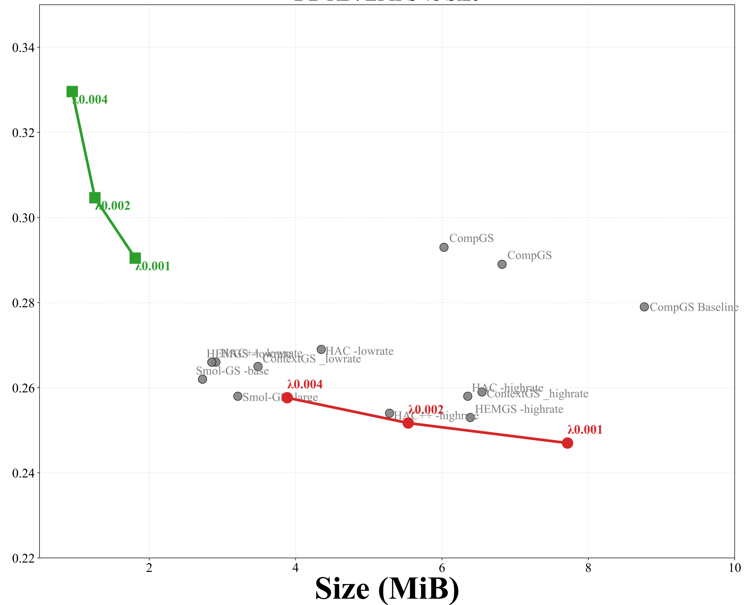
DB RD: LPIPS vs Size
