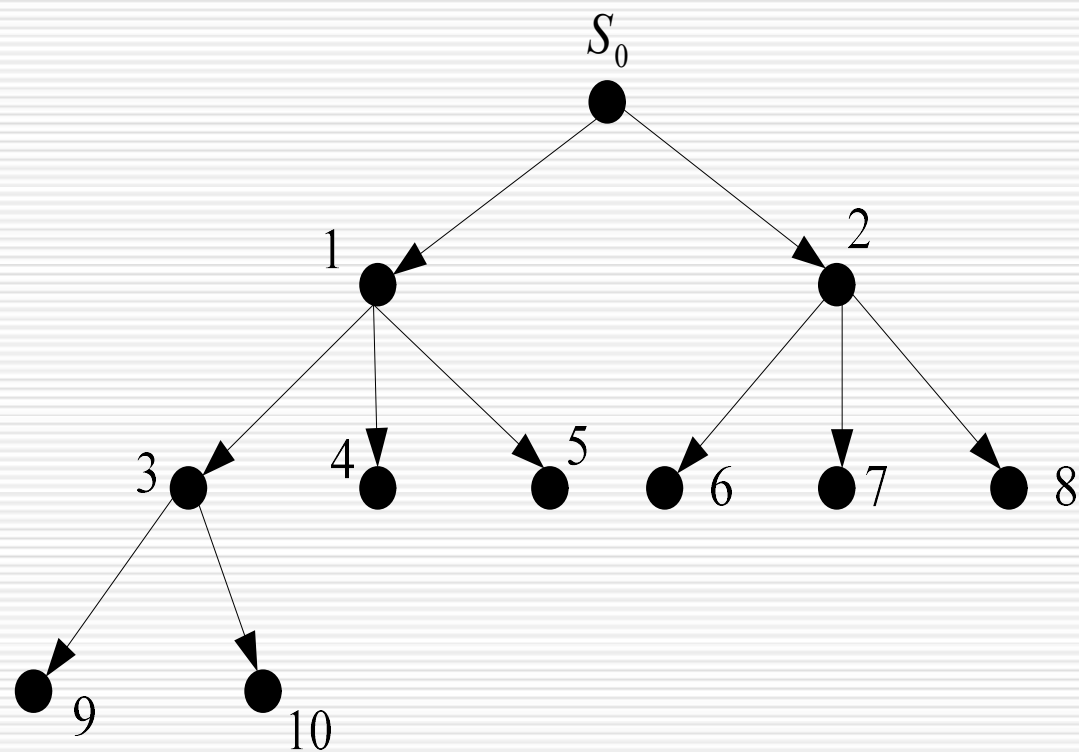
图5.6 宽度优先搜索法中状态的搜索次序
