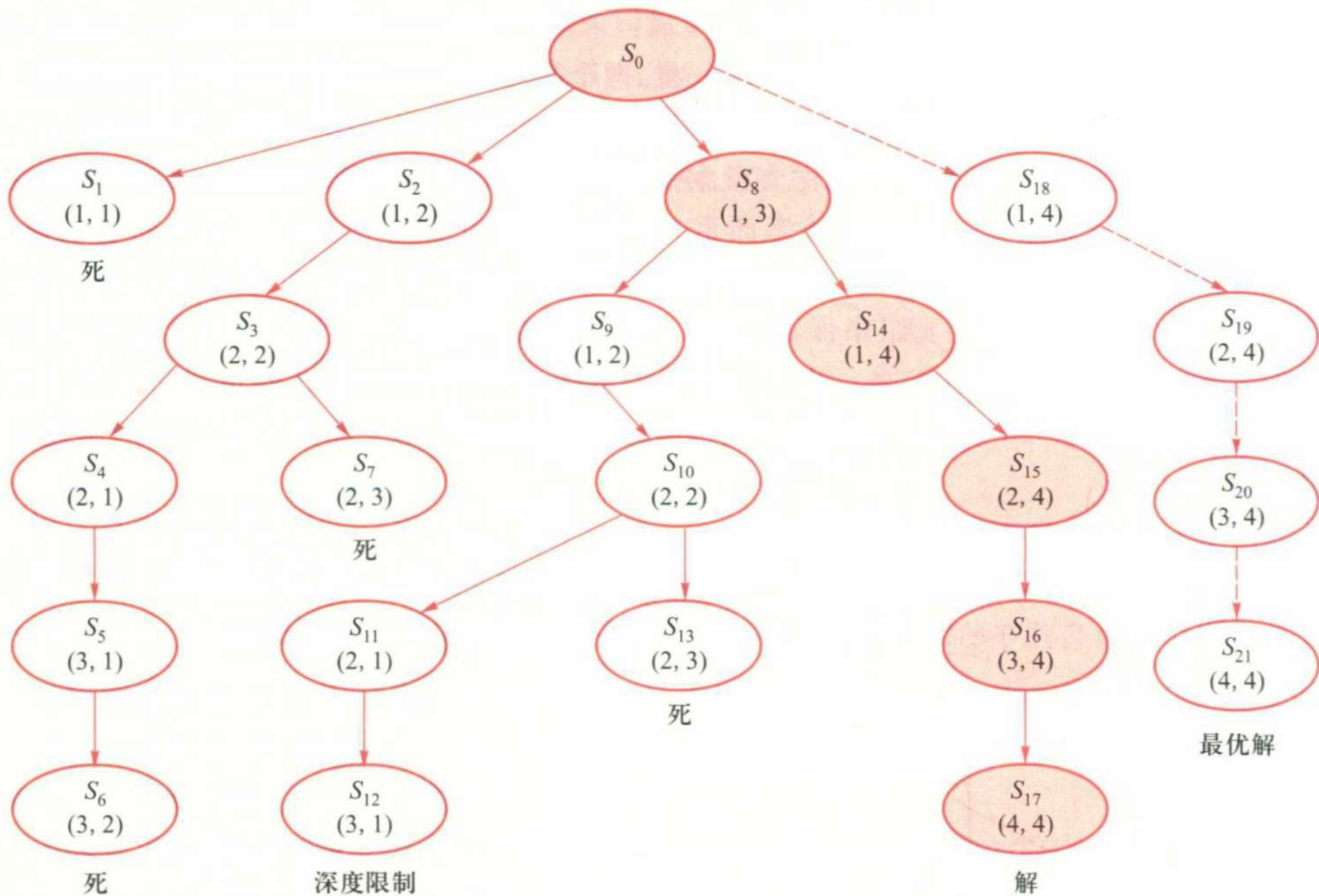
卒子穿阵的深度优先搜索树
