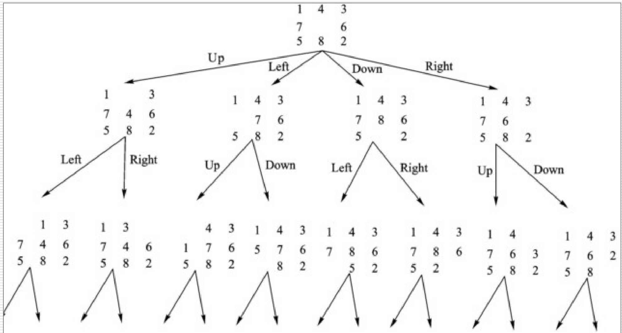
八数码状态空间图
