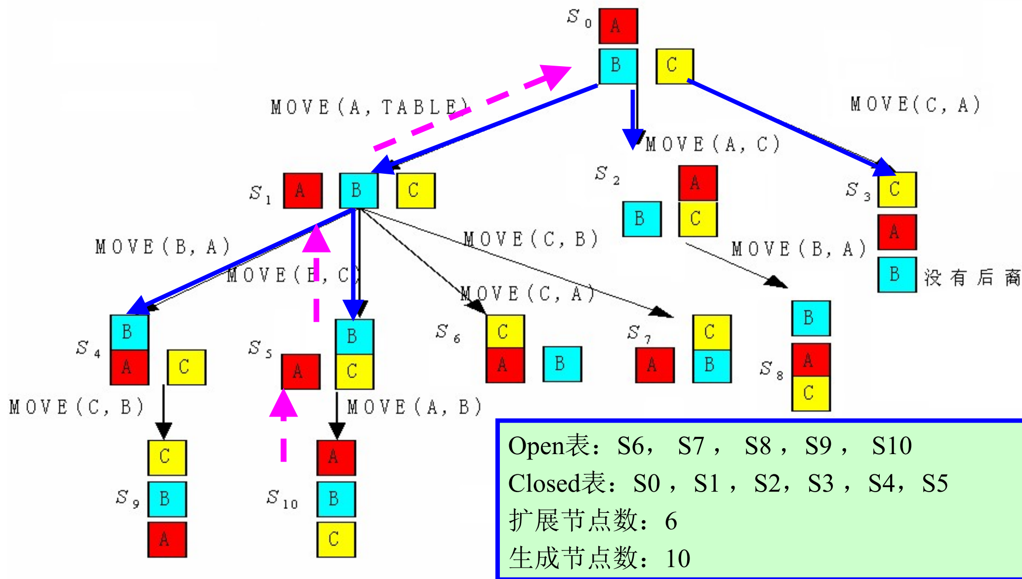
图 5.8 积木问题的宽度优先搜索树
