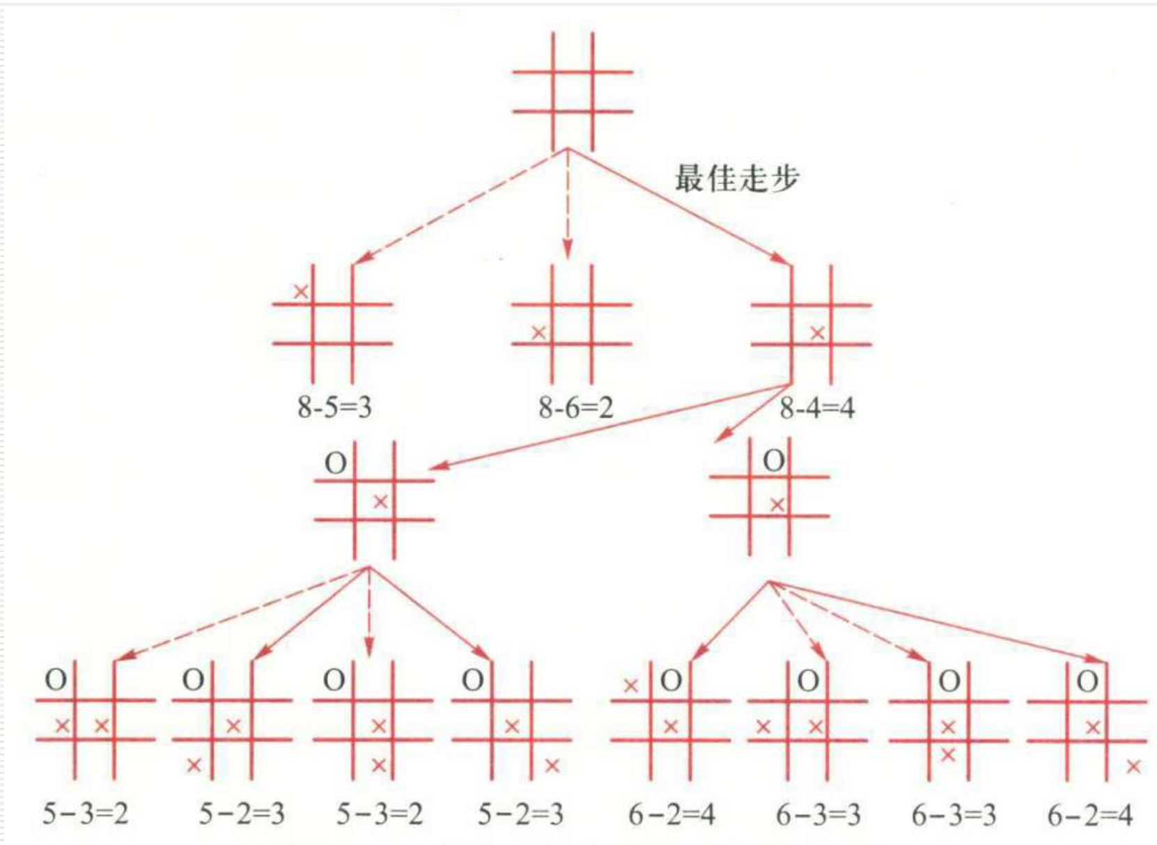
启发式搜索下缩减的状态空间
