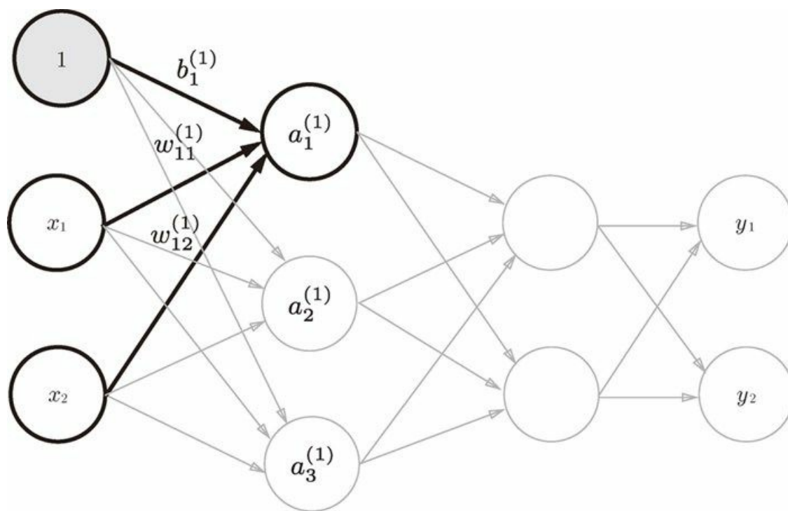
图 3-17 从输入层到第 1 层的信号传递
