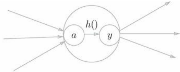
图 3-5 左图是一般的神经元的图，右图是在神经元内部明确显示激活函数的计算过程的图（ a 表示输入信号的总和， h() 表示激活函数， y 表示输出）
