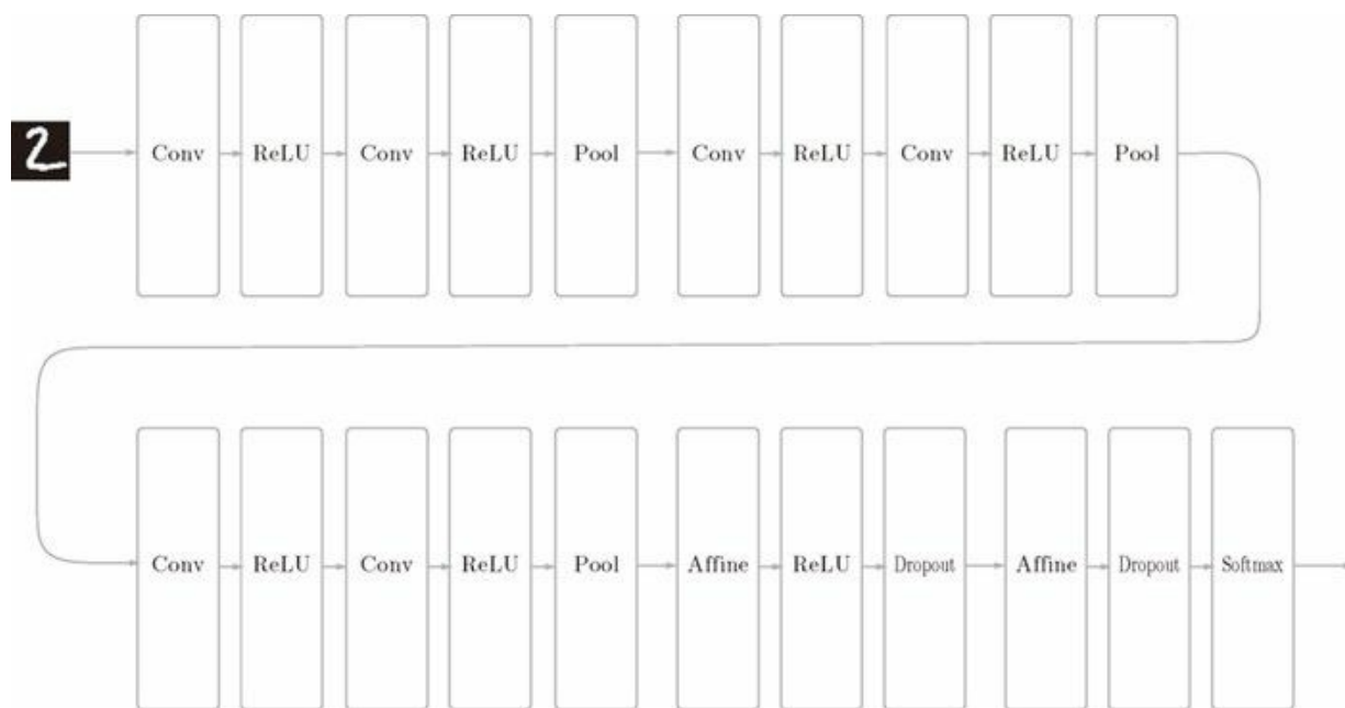
图 8-1 进行手写数字识别的深度 CNN
