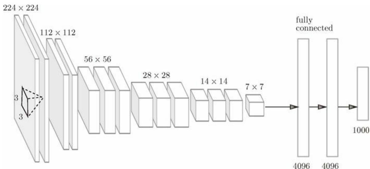
图 8-9 VGG（根据文献 [22] 生成）
