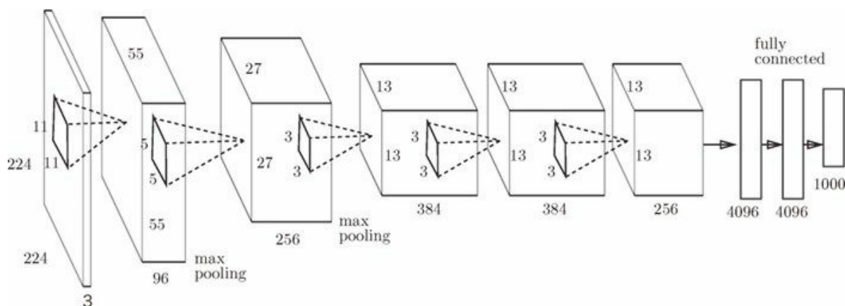
图 7-28 AlexNet（根据文献 [21] 生成）
