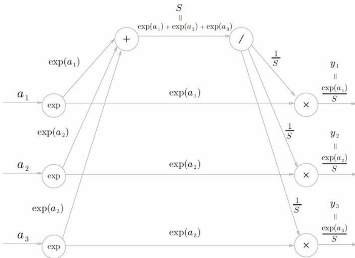
图 A-2 Softmax 层的计算图（仅正向传播）
