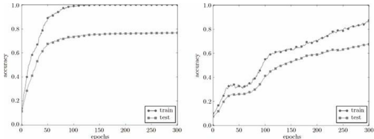
图 6-23 左边没有使用 Dropout ，右边使用了 Dropout （ dropout_rate=0.15 ）
