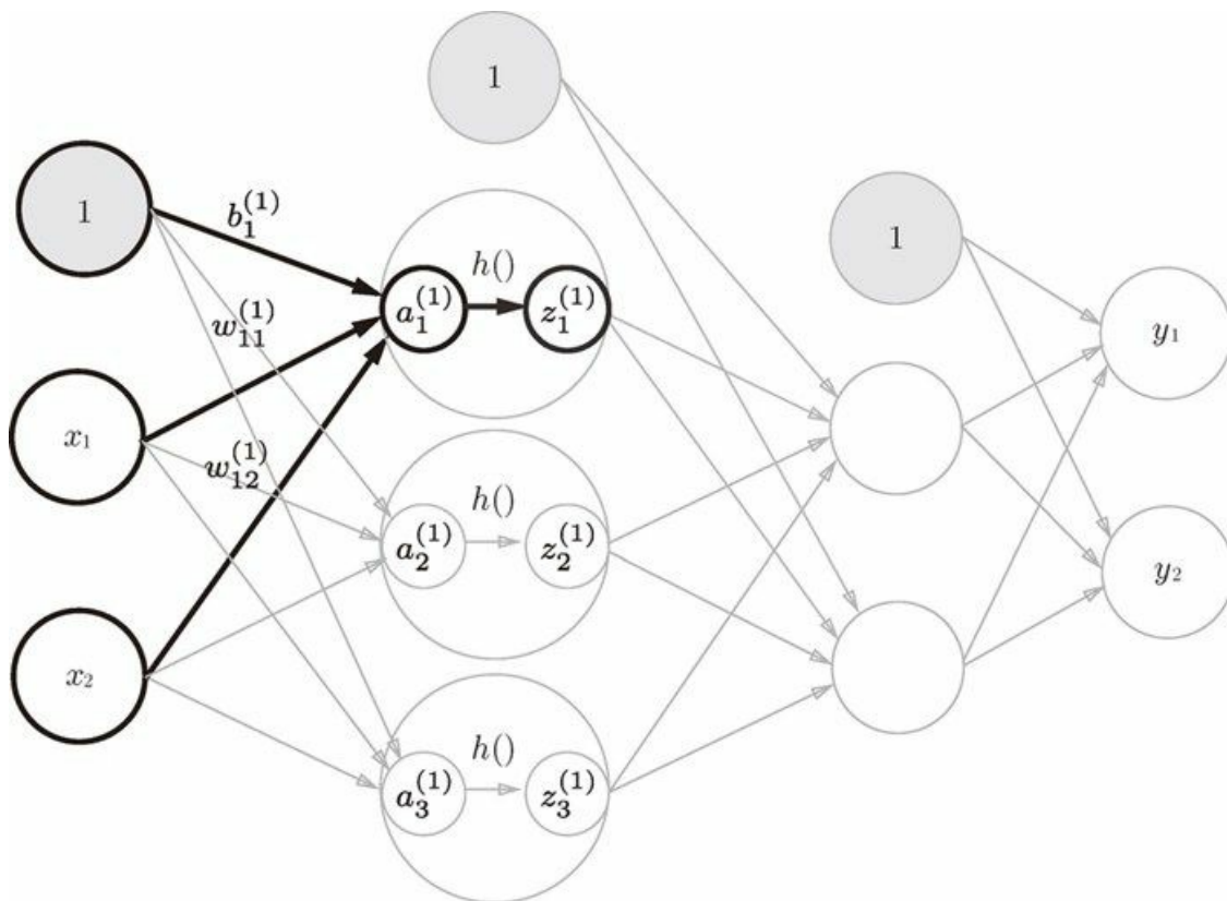
图 3-18 从输入层到第 1 层的信号传递
