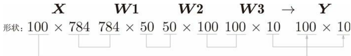
图 3-27 批处理中数组形状的变化
