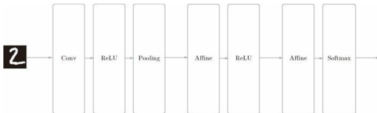
图 7-23 简单 CNN 的网络构成
