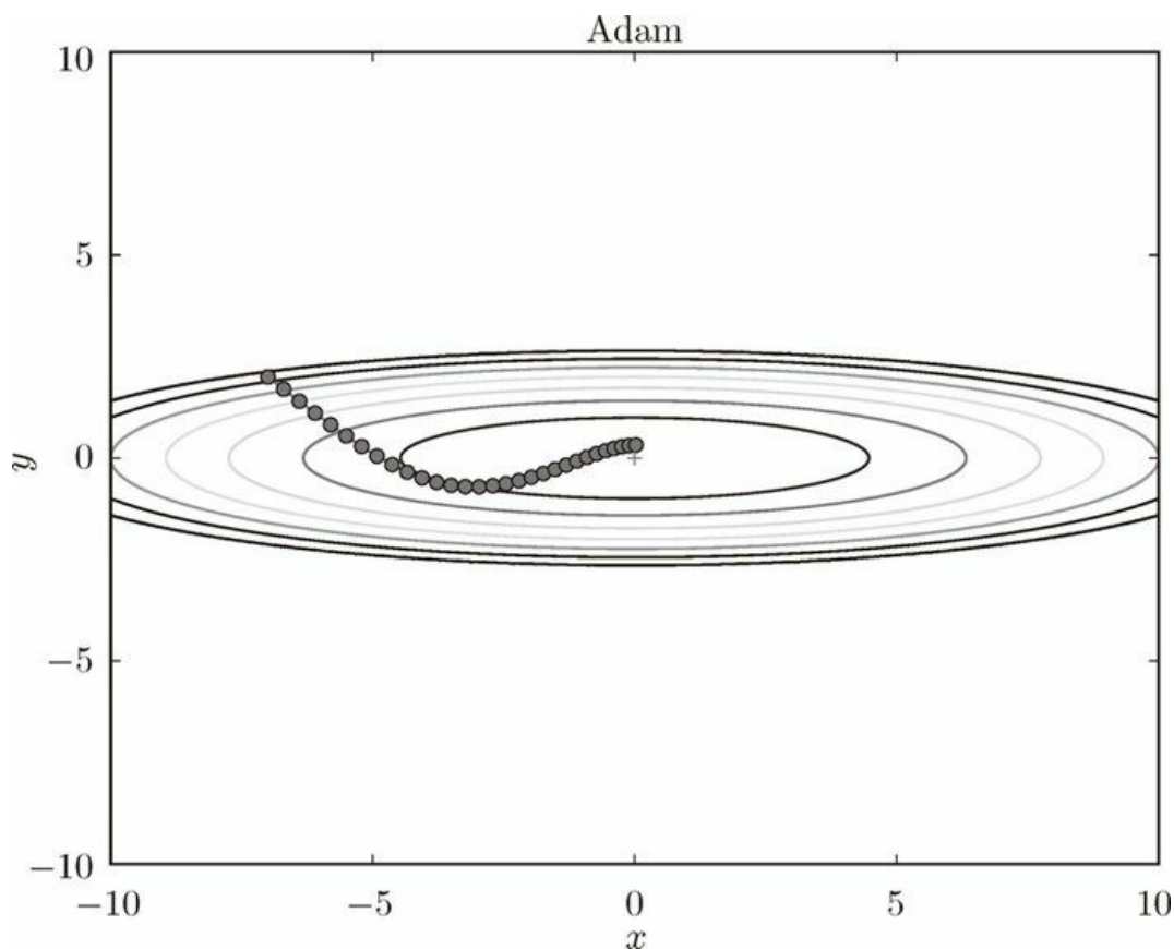
图 6-7 基于 Adam 的最优化的更新路径
