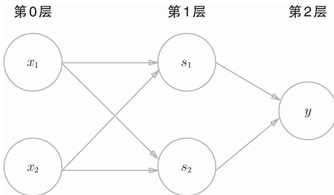
图 2-13 用感知机表示异或门
