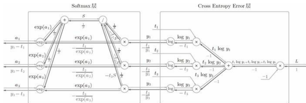
图 A-5 Softmax-with-Loss 层的计算图
