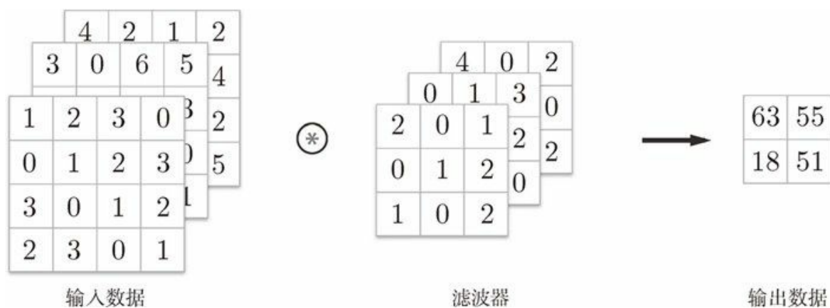
图 7-8 对 3 维数据进行卷积运算的例子
