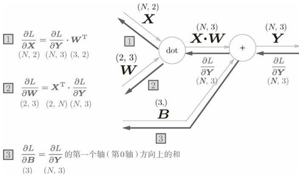
图 5-27 批版本的 Affine 层的计算图
