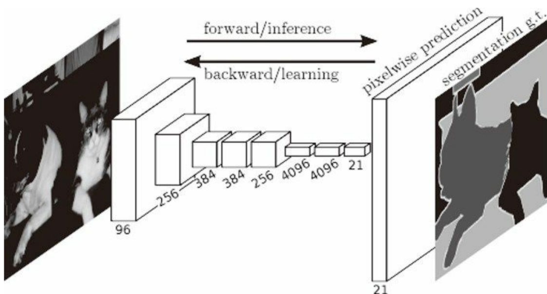
图 8-20 FCN 的概略图（引用自文献 [37]）
