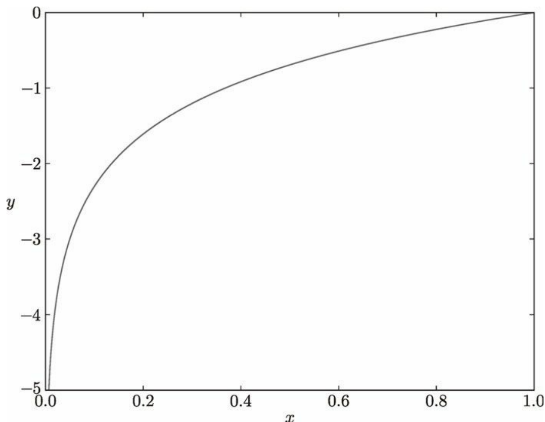
图 4-3 自然对数 y = \log x 的图像
