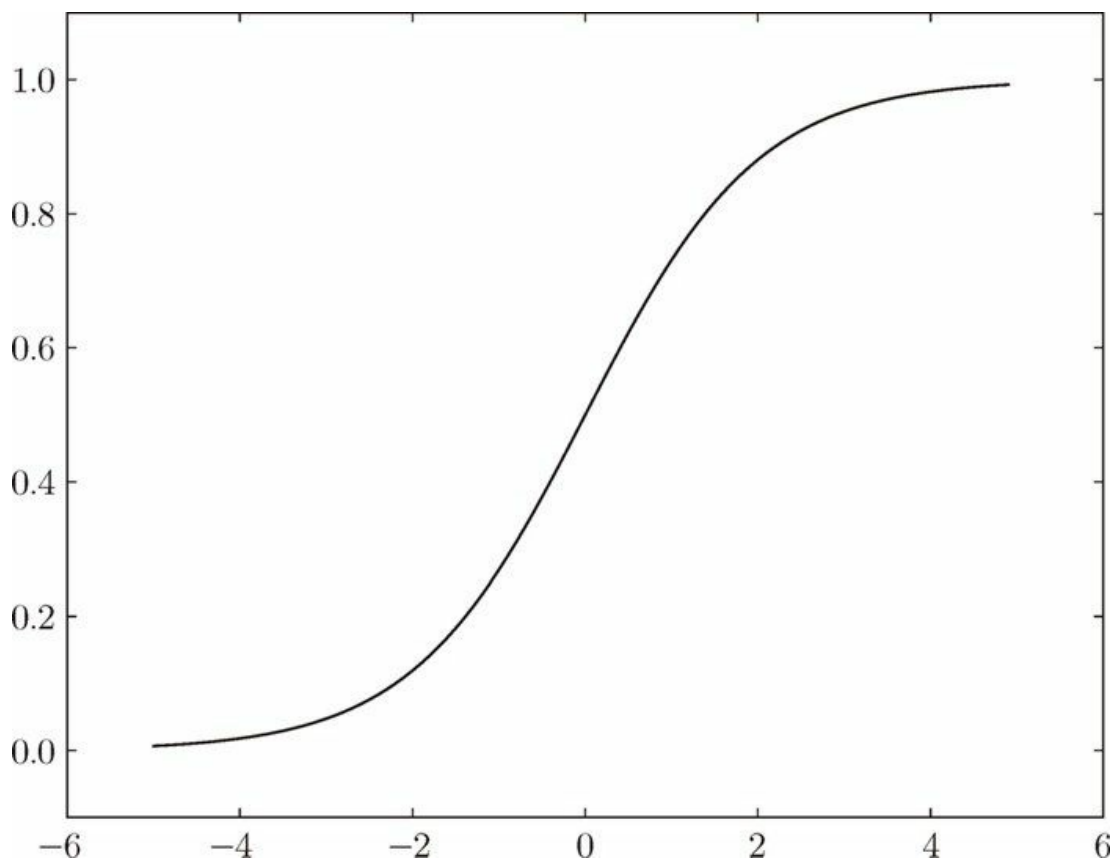
图 3-7 sigmoid 函数的图形
