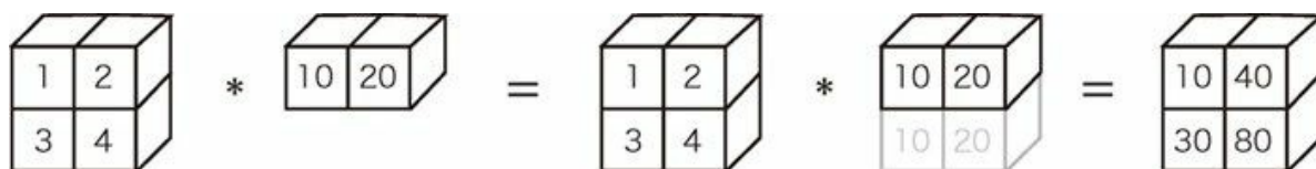
图 1-2 广播的例子 2
