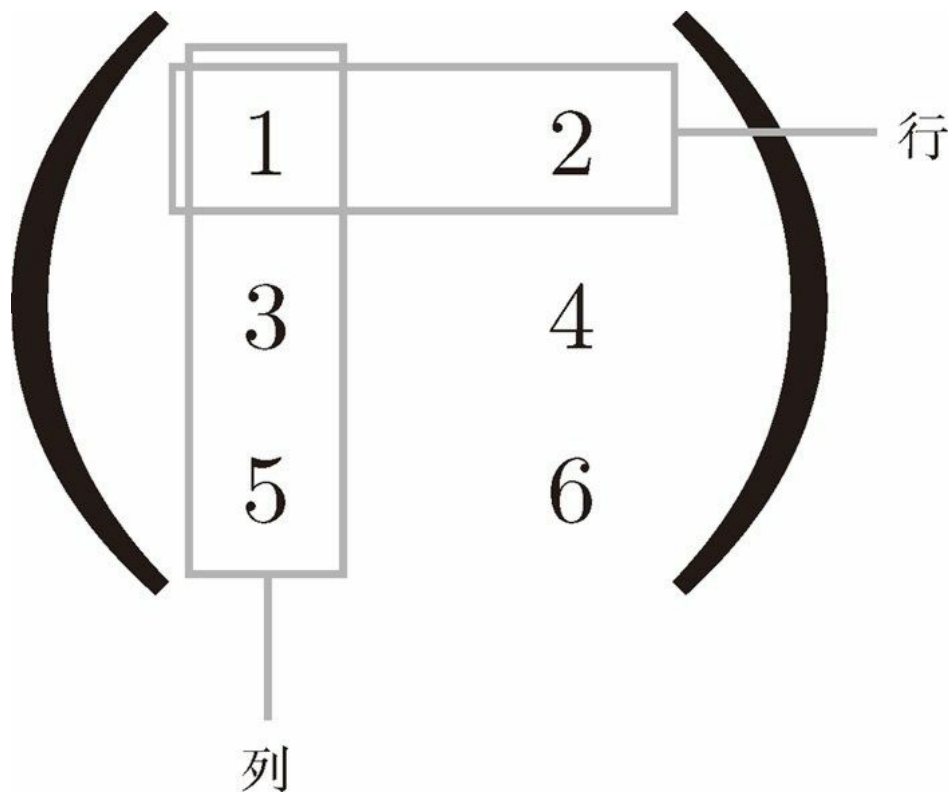
图 3-10 横向排列称为行，纵向排列称为列
