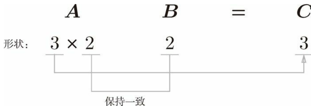
图 3-13 A 是二维矩阵、 B 是一维数组时，也要保持对应维度的元素个数一致
