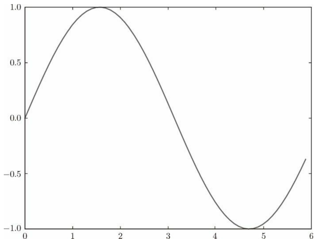
图 1-3 sin 函数的图形
