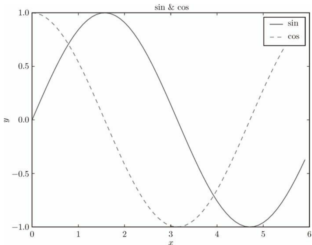
图 1-4 sin 函数和 cos 函数的图形
