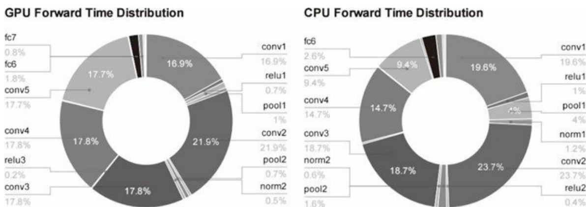
图 8-14 AlexNet 的 forward 处理中各层的时间比：左边是使用 GPU 的情况，右边是使用 CPU 的情况。图中的“conv”对应卷积层，“pool”对应池化层，“fc”对应全连接层，“norm”对应正规化层（引用自文献 [26]）
