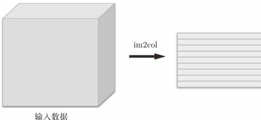
图 7-17 im2col 的示意图
