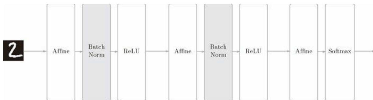
图 6-16 使用了 Batch Normalization 的神经网络的例子（Batch Norm 层的背景为灰色）
