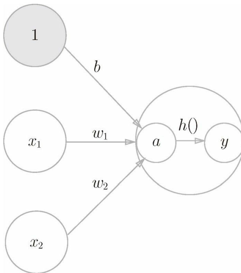
图 3-4 明确显示激活函数的计算过程
