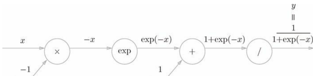
图 5-19 sigmoid 层的计算图（仅正向传播）
