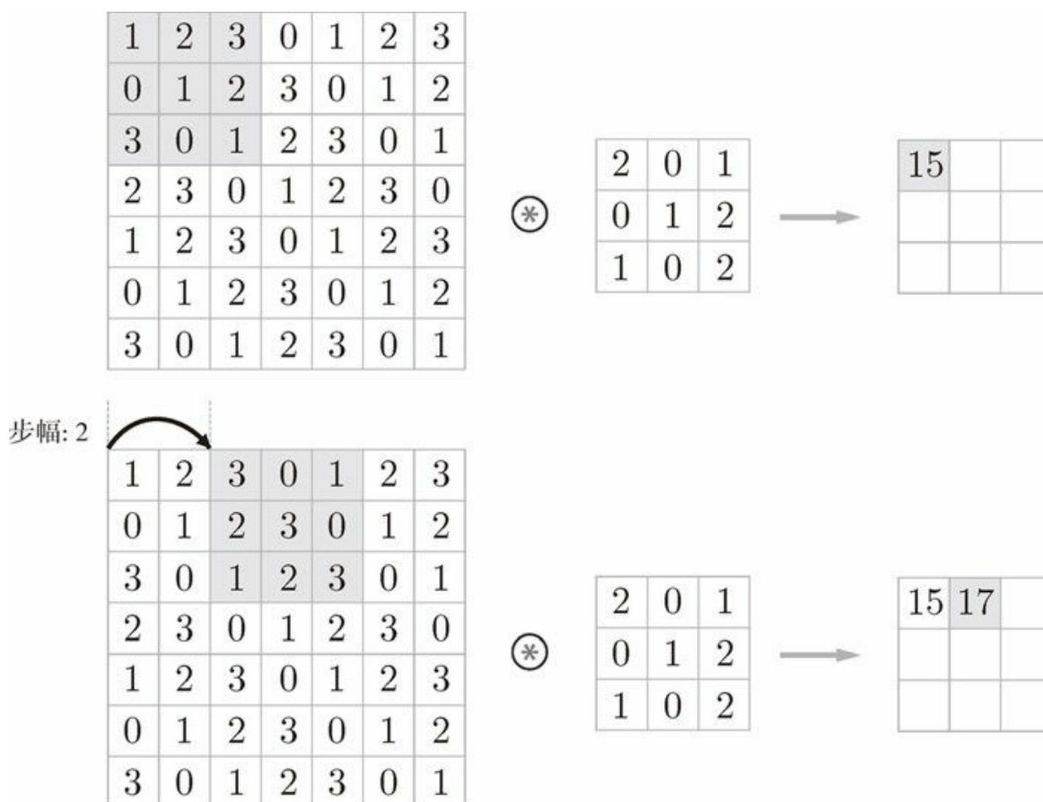
图 7-7 步幅为 2 的卷积运算的例子
