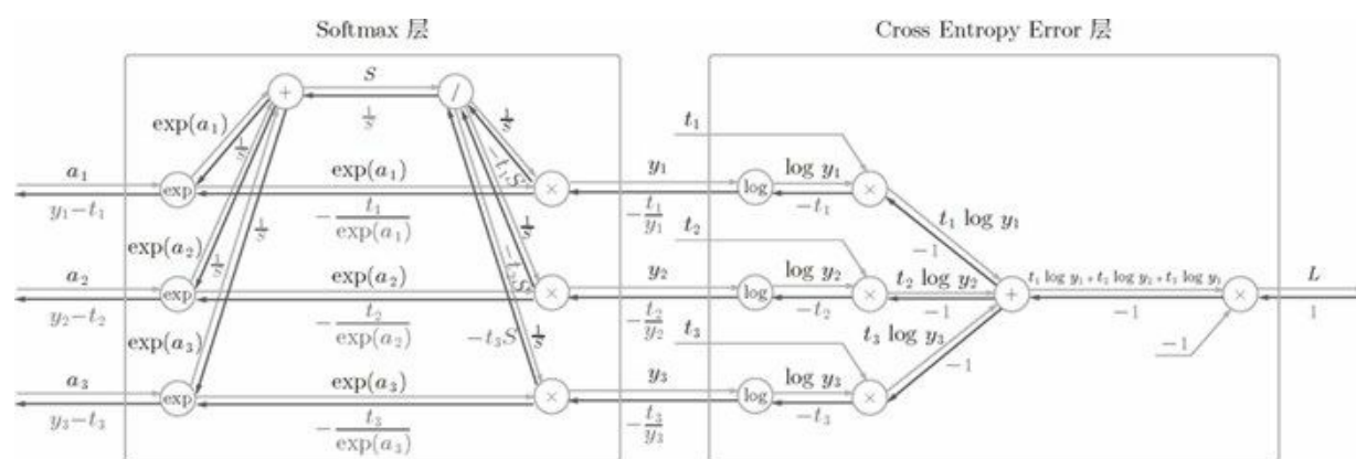
图 5-29 Softmax-with-Loss 层的计算图
