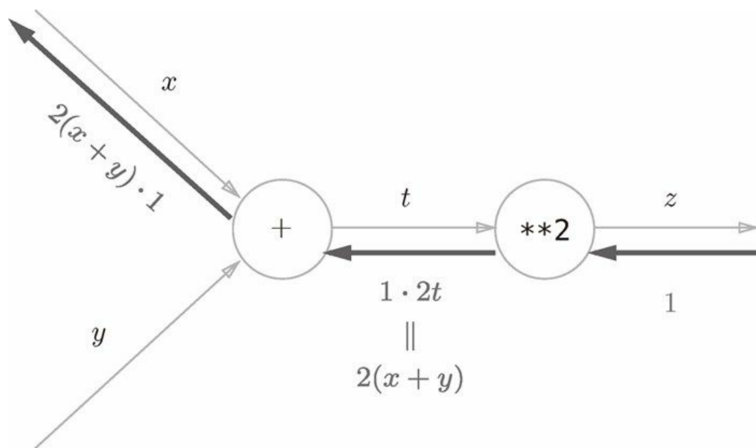
图 5-8 根据计算图的反向传播的结果， \frac{\partial z}{\partial x} 等于 2(x+y)
