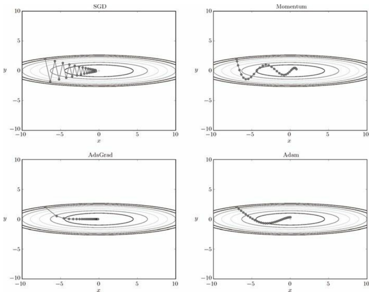
图 6-8 最优化方法的比较：SGD、Momentum、AdaGrad、Adam
