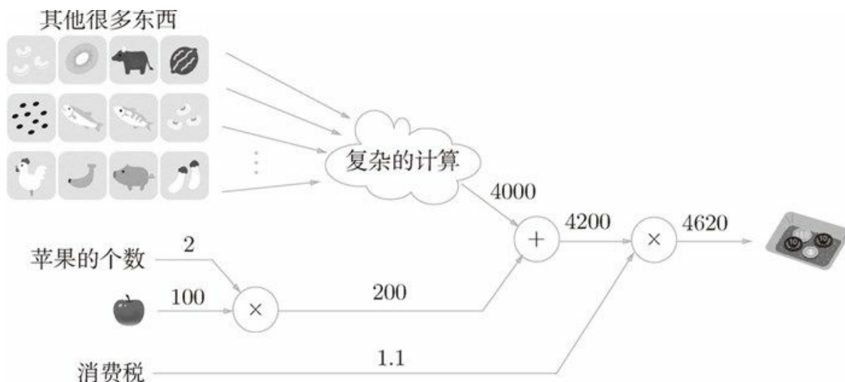
图 5-4 买了 2 个苹果和其他很多东西的例子
