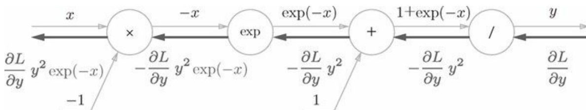
图 5-20 Sigmoid 层的计算图
