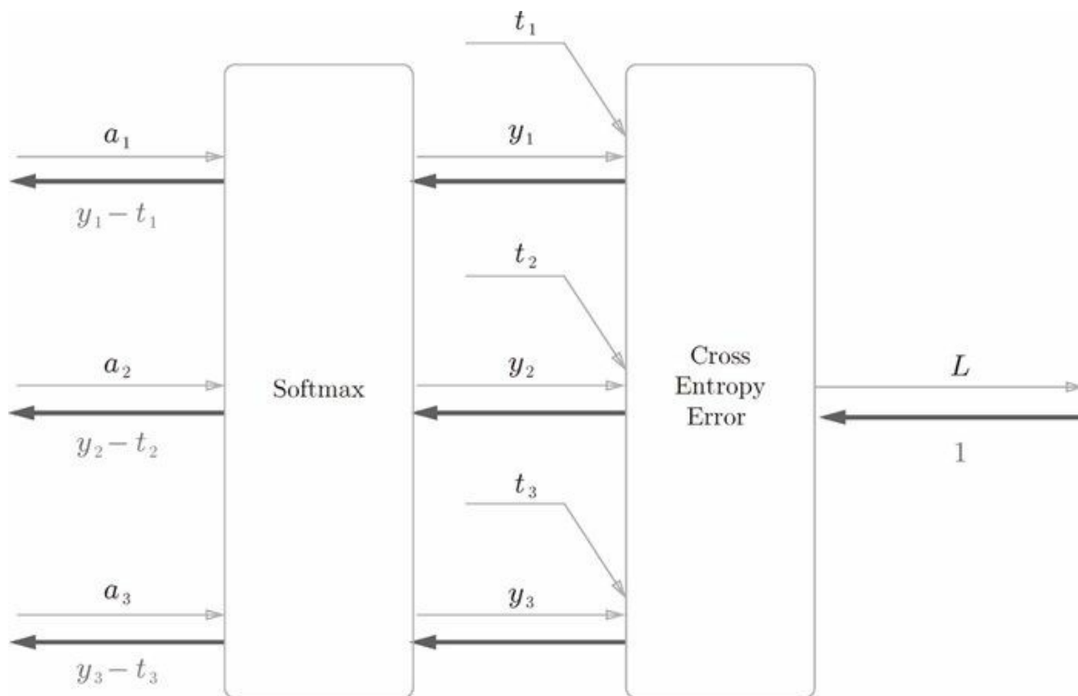
图 A-1 Softmax-with-Loss 层的计算图
