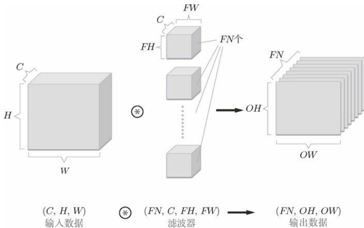
图 7-11 基于多个滤波器的卷积运算的例子
