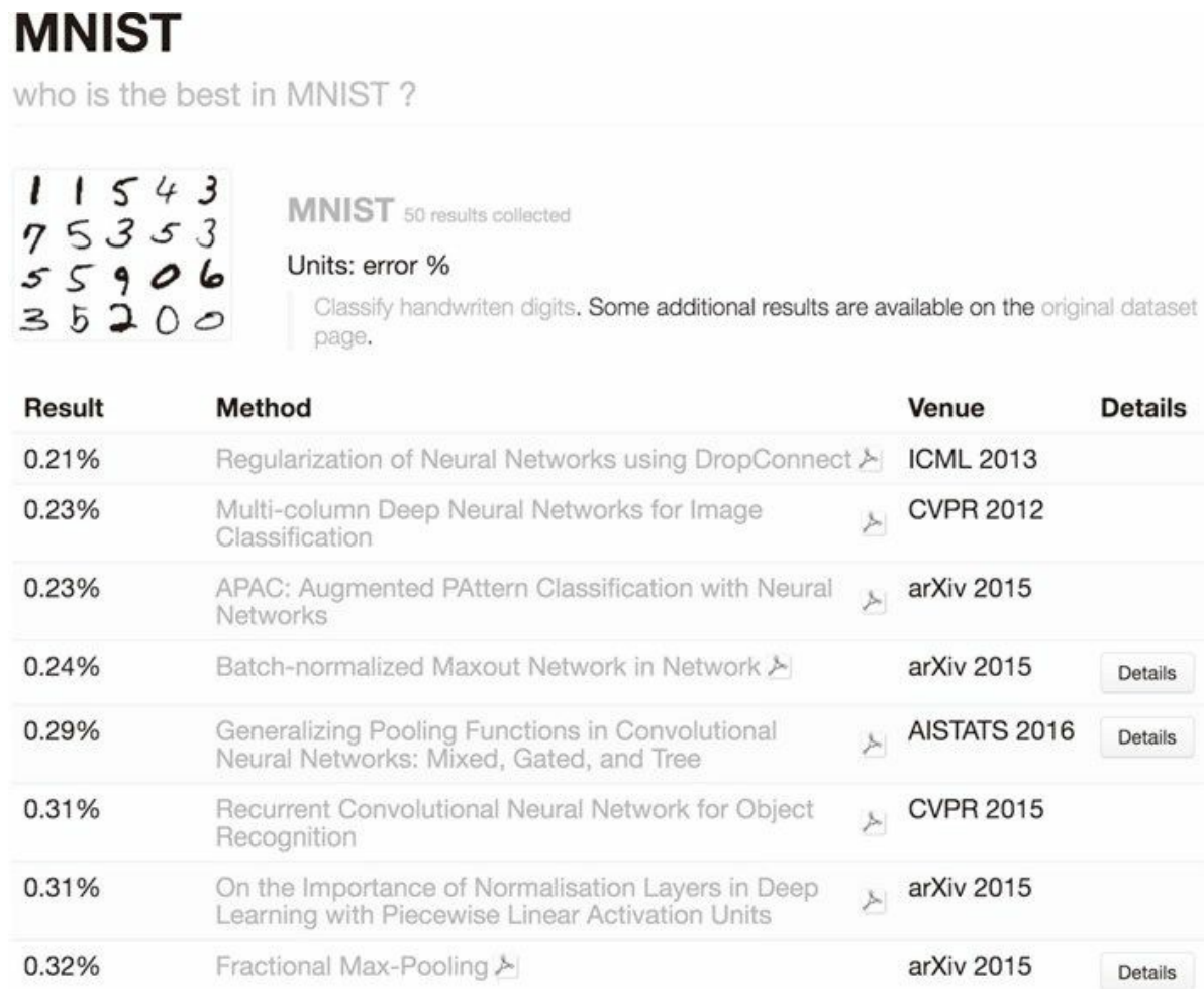
图 8-3 针对 MNIST 数据集的各种方法的排行（引自文献 [32]：2016 年 6 月）
