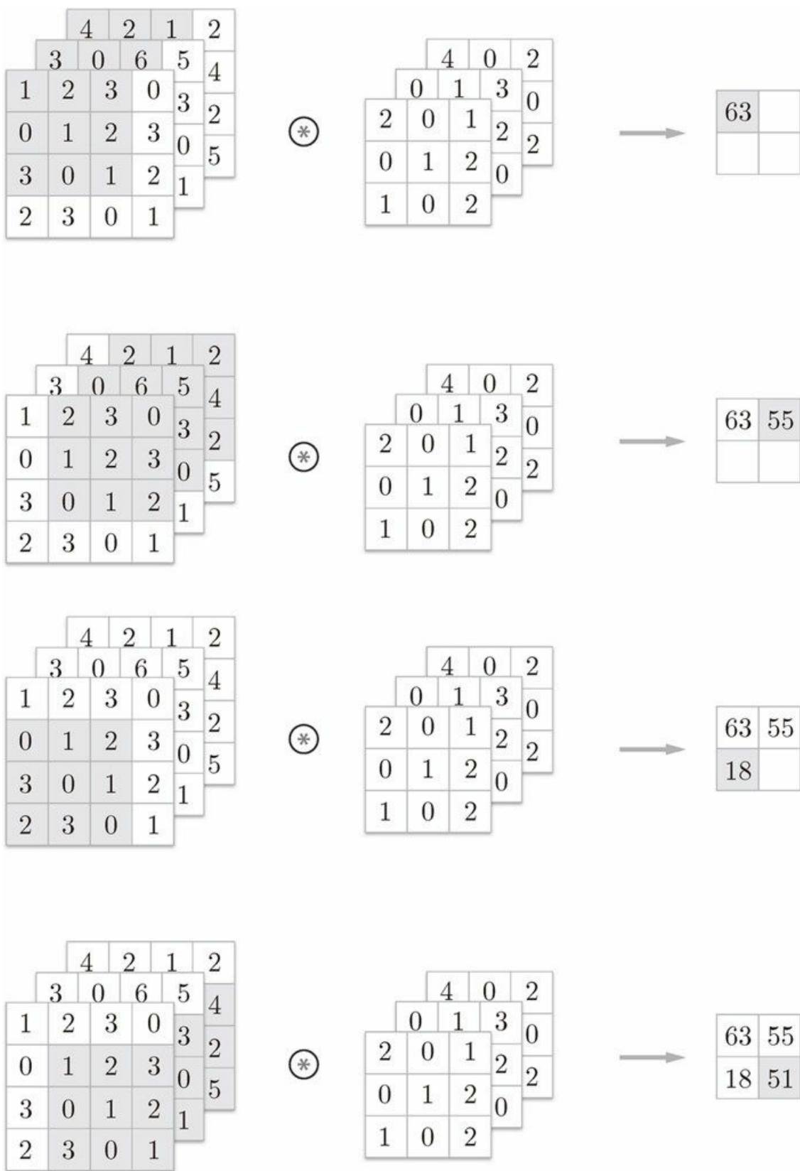
图 7-9 对 3 维数据进行卷积运算的计算顺序
