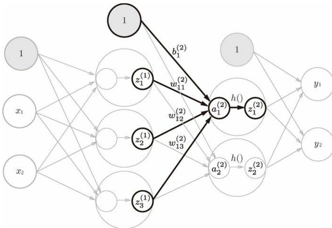
图 3-19 第 1 层到第 2 层的信号传递
