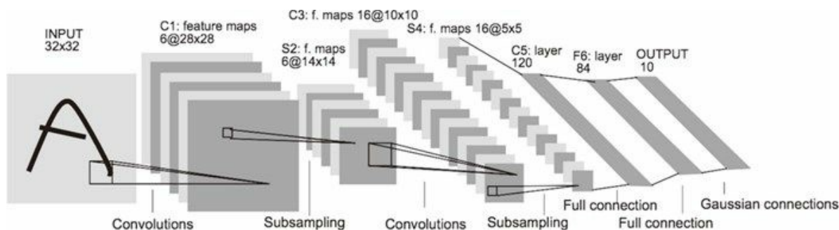
图 7-27 LeNet 的网络结构（引用自文献 [20]）
