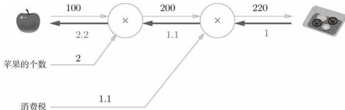
图 5-5 基于反向传播的导数的传递
