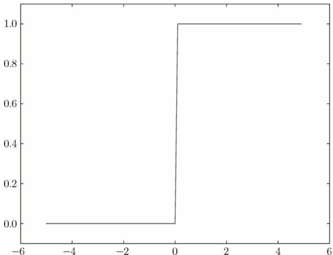
图 3-6 阶跃函数的图形
