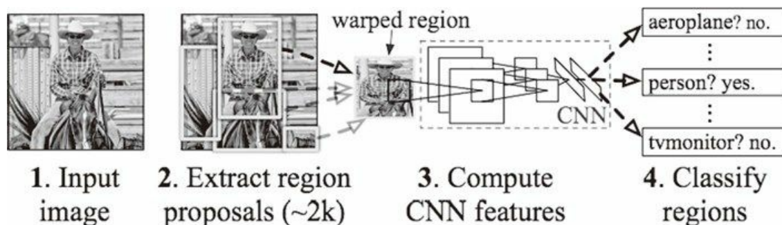
图 8-18 R-CNN 的处理流（引用自文献 [35]）
