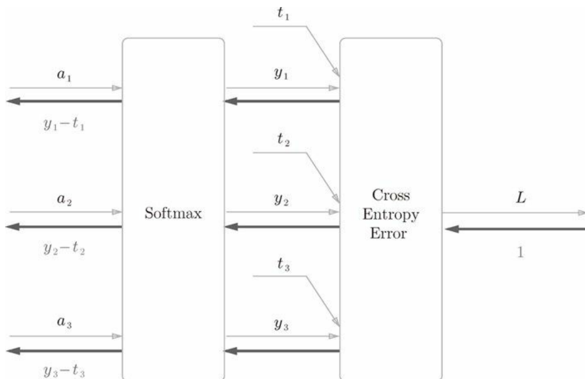
图 5-30 “简易版”的 Softmax-with-Loss 层的计算图
