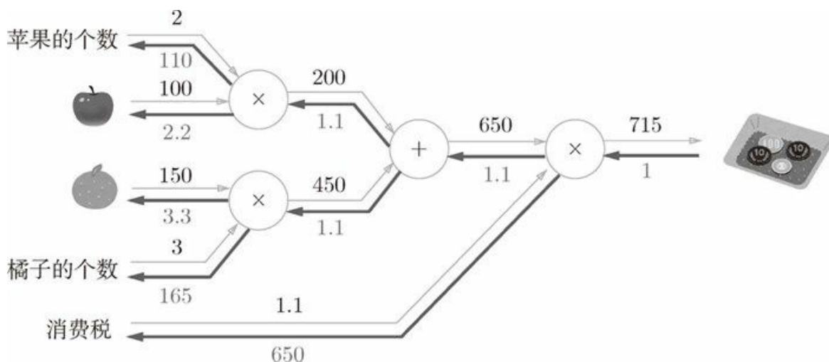
图 5-17 购买 2 个苹果和 3 个橘子
