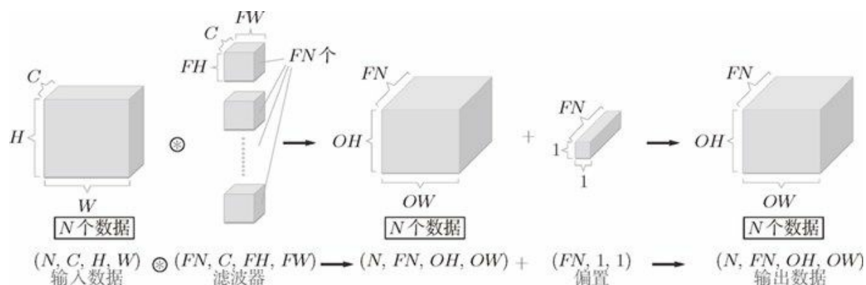
图 7-13 卷积运算的处理流（批处理）
