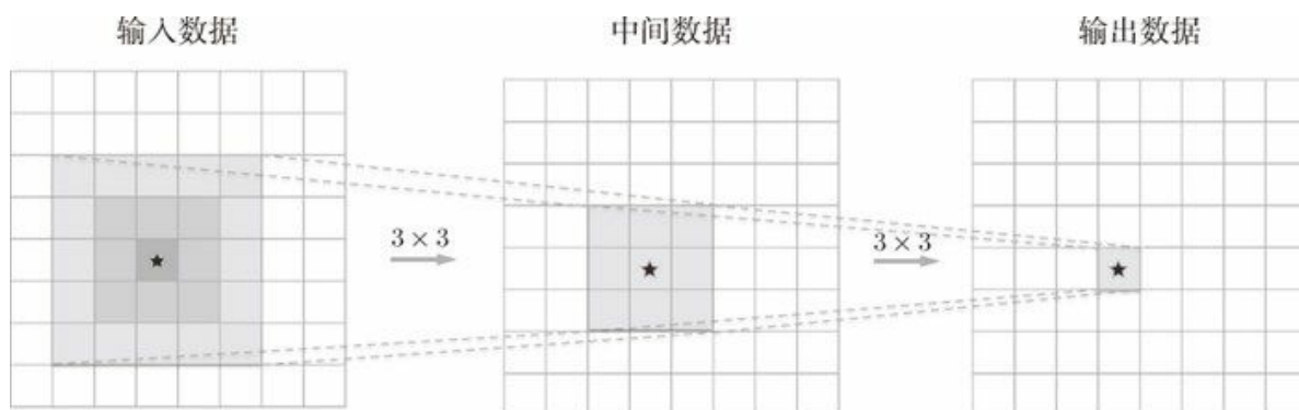
图 8-6 重复两次 3 \times 3 的卷积层的例子
