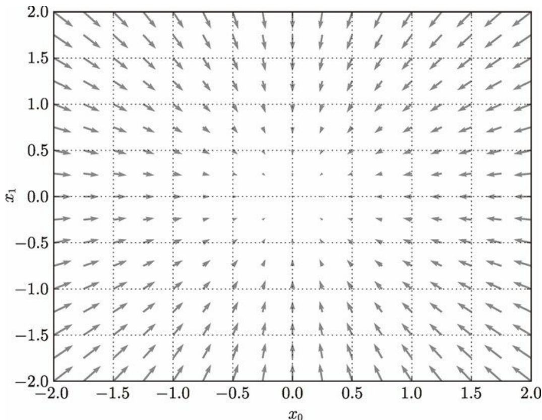
图 4-9 f(x_0, x_1) = x_0^2 + x_1^2 的梯度
