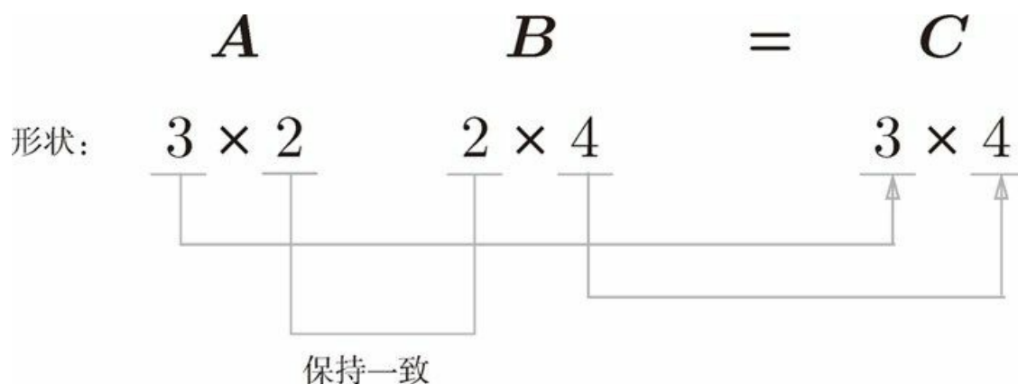
图 3-12 在矩阵的乘积运算中，对应维度的元素个数要保持一致
