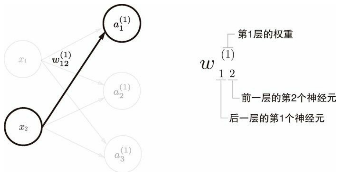
图 3-16 权重的符号
