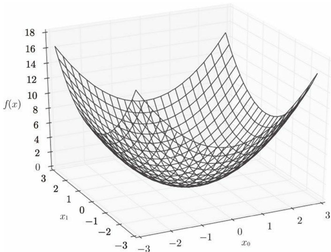
图 4-8 f(x_0, x_1) = x_0^2 + x_1^2 的图像
