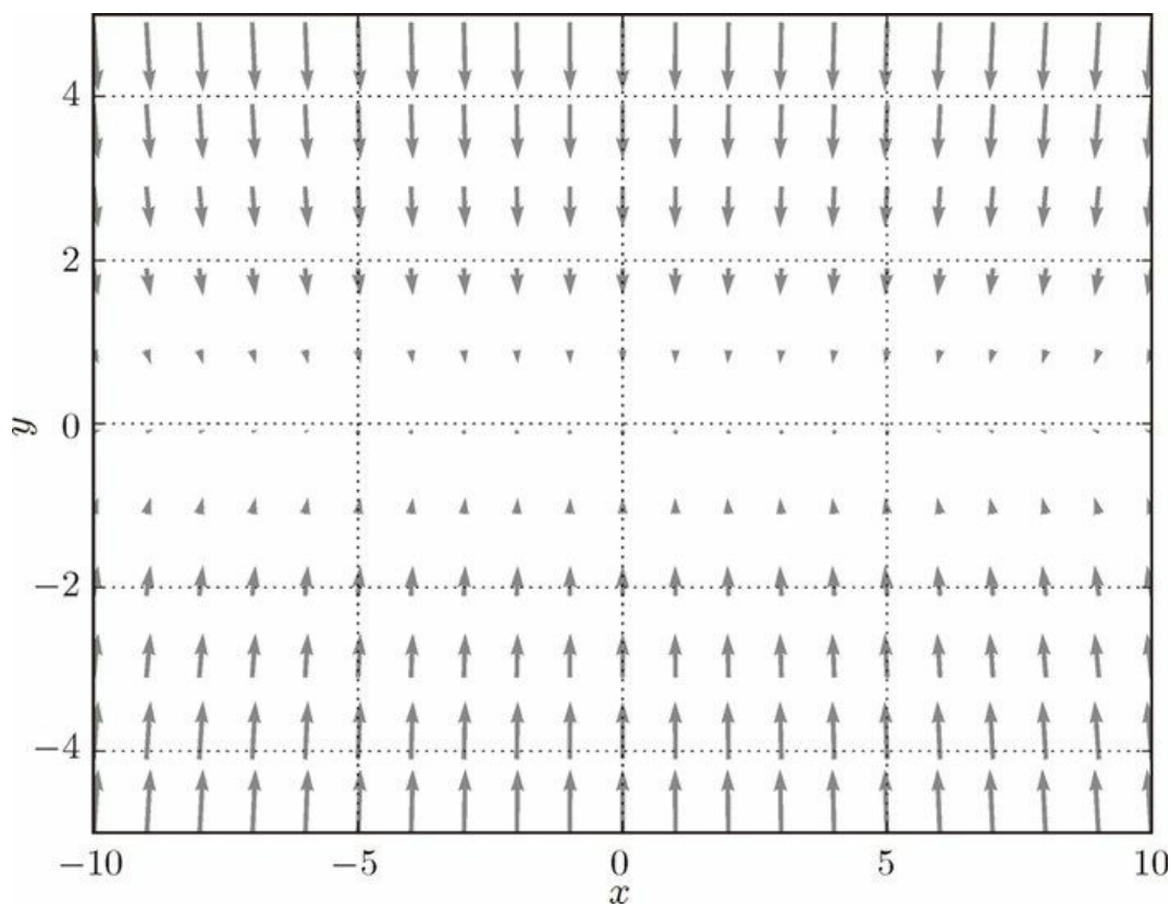
图 6-2 f(x, y) = \frac{1}{20}x^2 + y^2 的梯度
