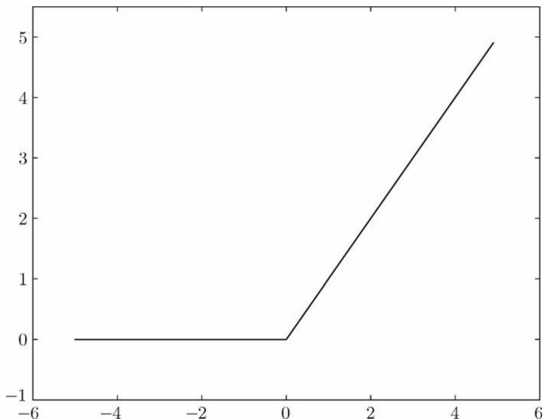
图 3-9 ReLU 函数
