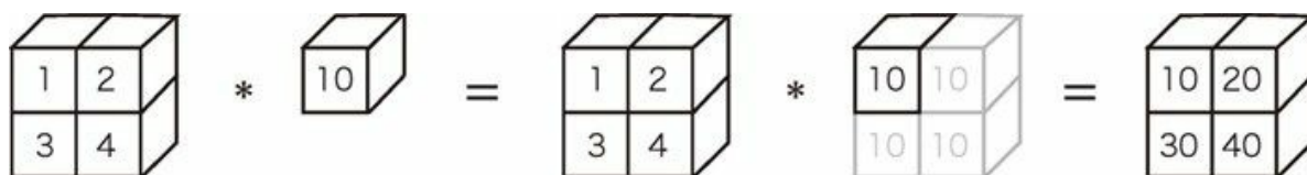
图 1-1 广播的例子：标量 10 被当作 2 \times 2 的矩阵
