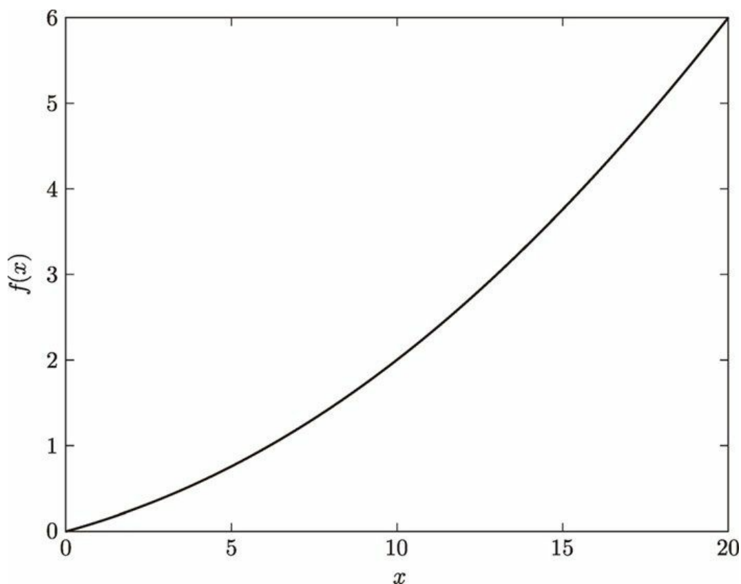
图 4-6 f(x) = 0.01x^2 + 0.1x 的图像
