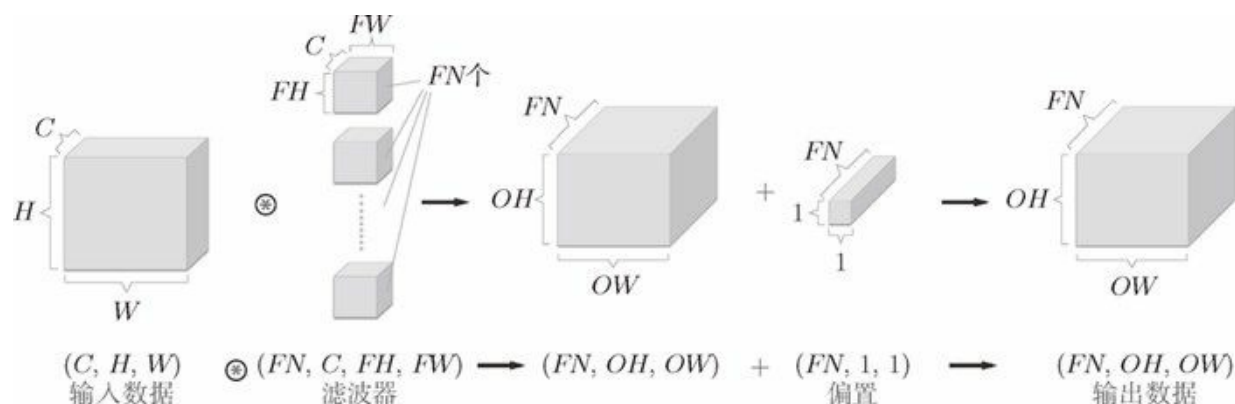
图 7-12 卷积运算的处理流（追加了偏置项）
