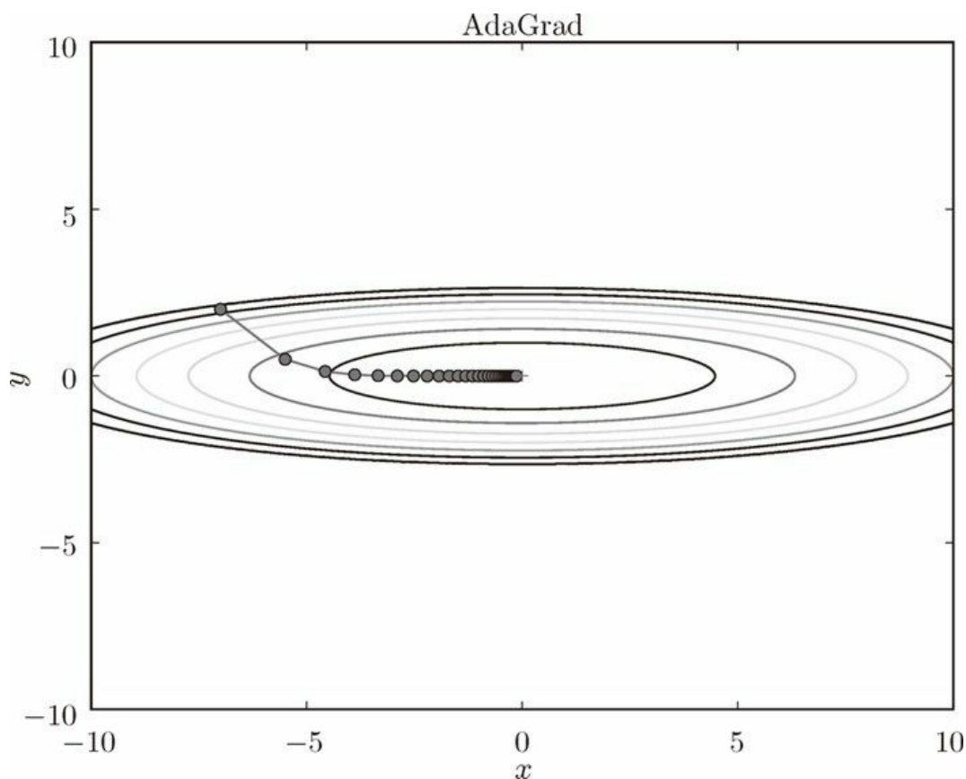
图 6-6 基于 AdaGrad 的最优化的更新路径
