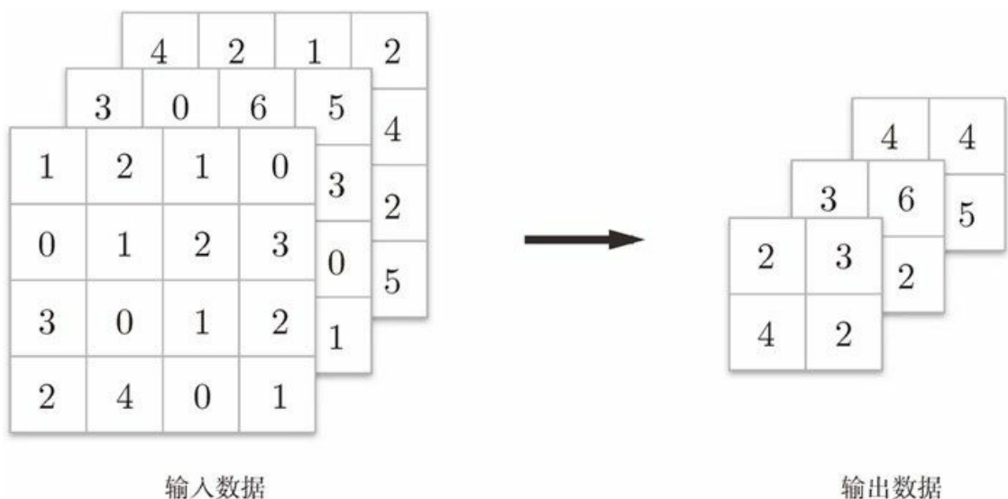
图 7-15 池化中通道数不变
