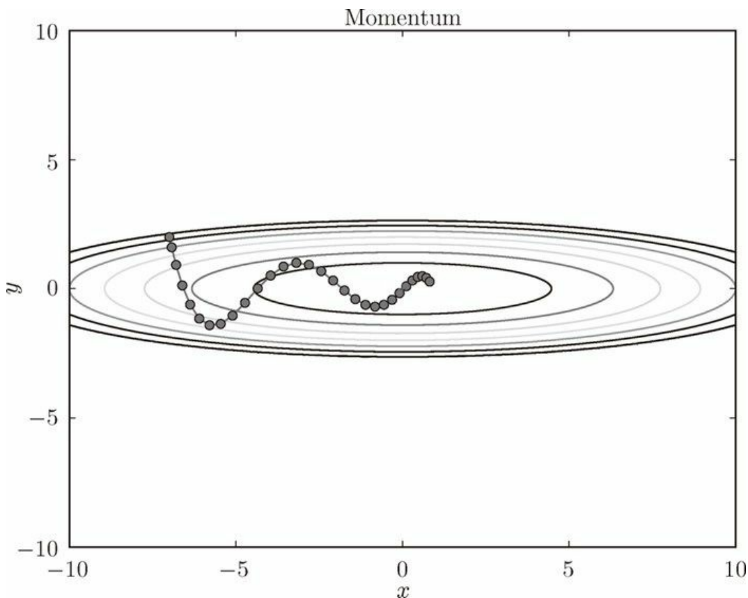
图 6-5 基于 Momentum 的最优化的更新路径
