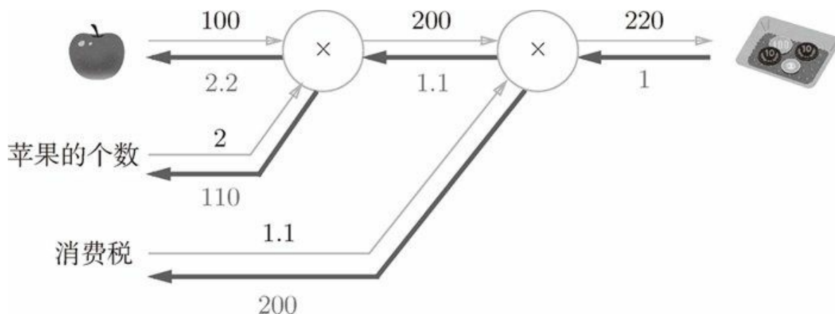
图 5-14 购买苹果的反向传播的例子
