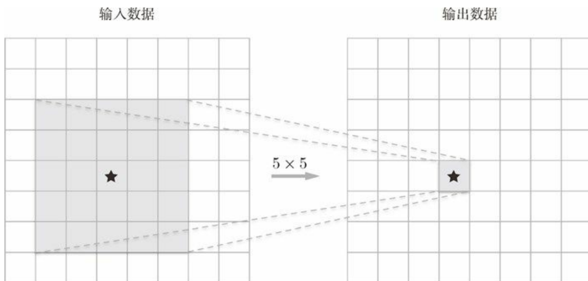
图 8-5 5 \times 5 的卷积运算的例子
