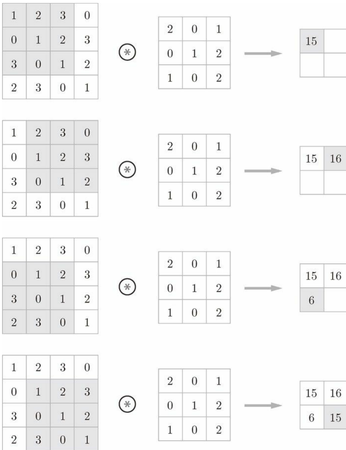
图 7-4 卷积运算的计算顺序
