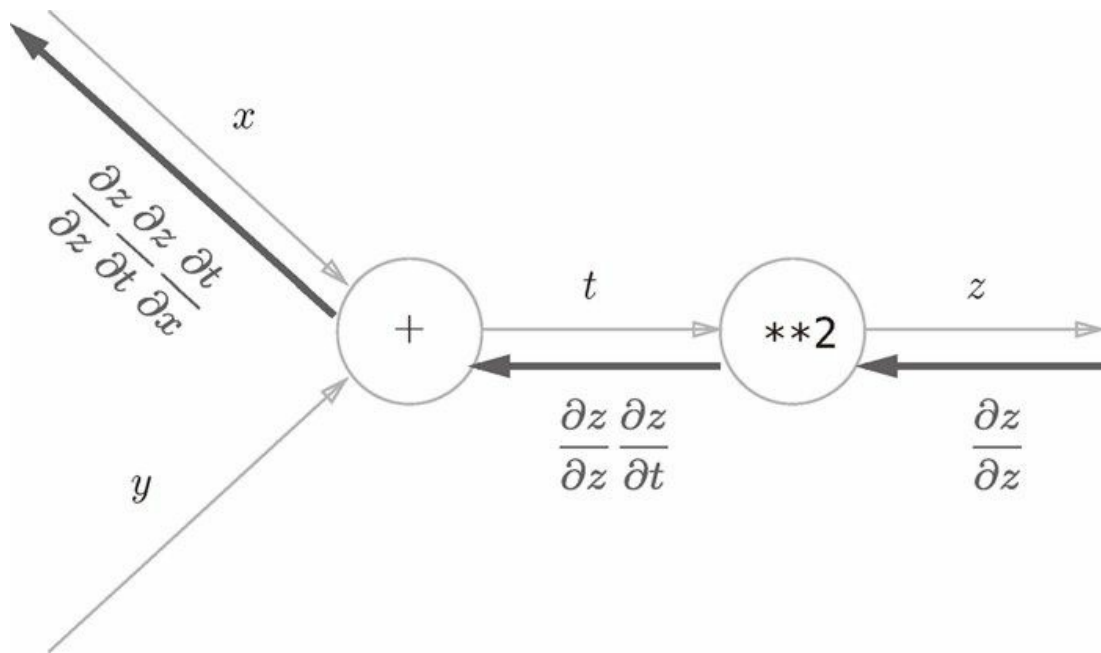
图 5-7 式 (5.4) 的计算图：沿着与正方向相反的方向，乘上局部导数后传递
