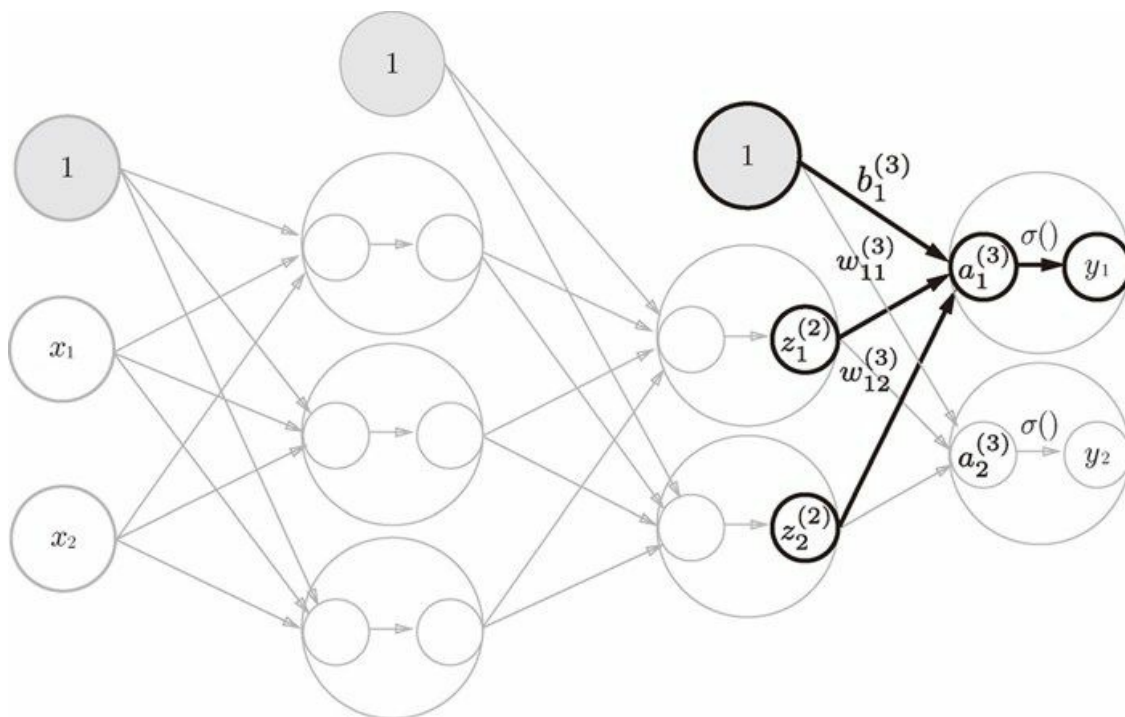
图 3-20 从第 2 层到输出层的信号传递
