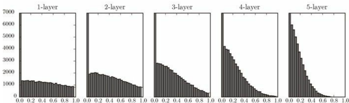
权重初始值为 Xavier 初始值时
