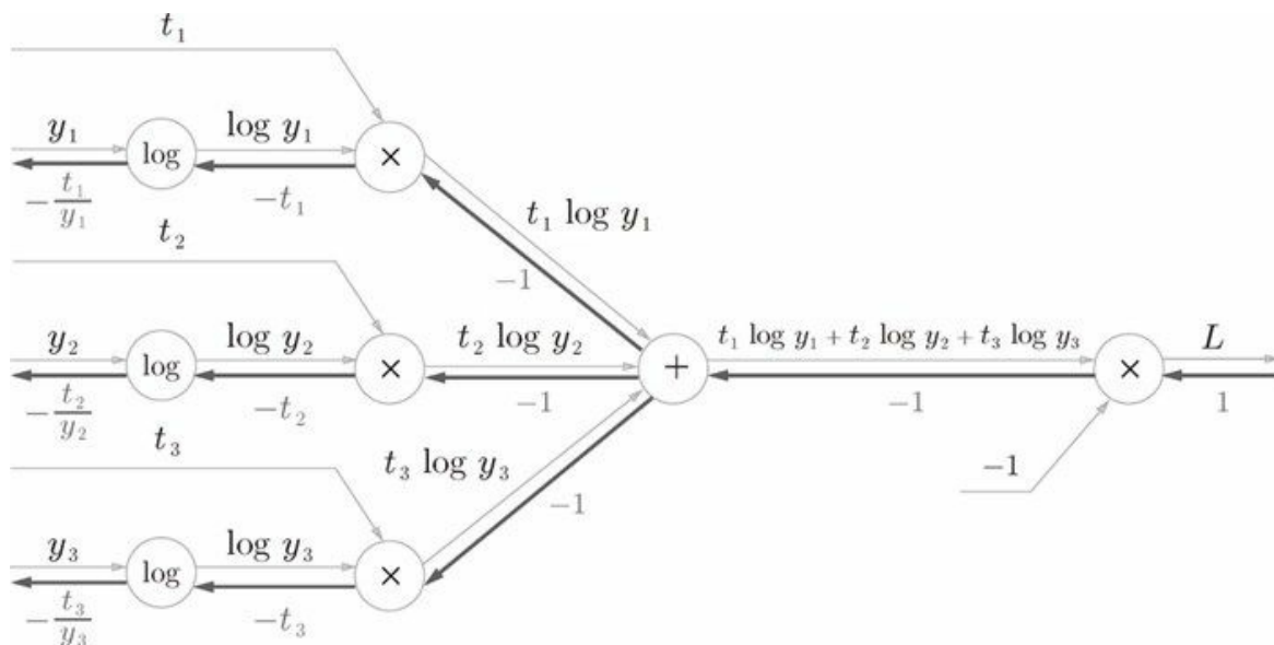
图 A-4 交叉熵误差的反向传播
