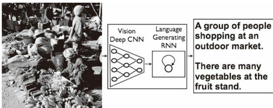
图 8-22 Neural Image Caption（NIC）的整体结构（引用自文献 [38]）
