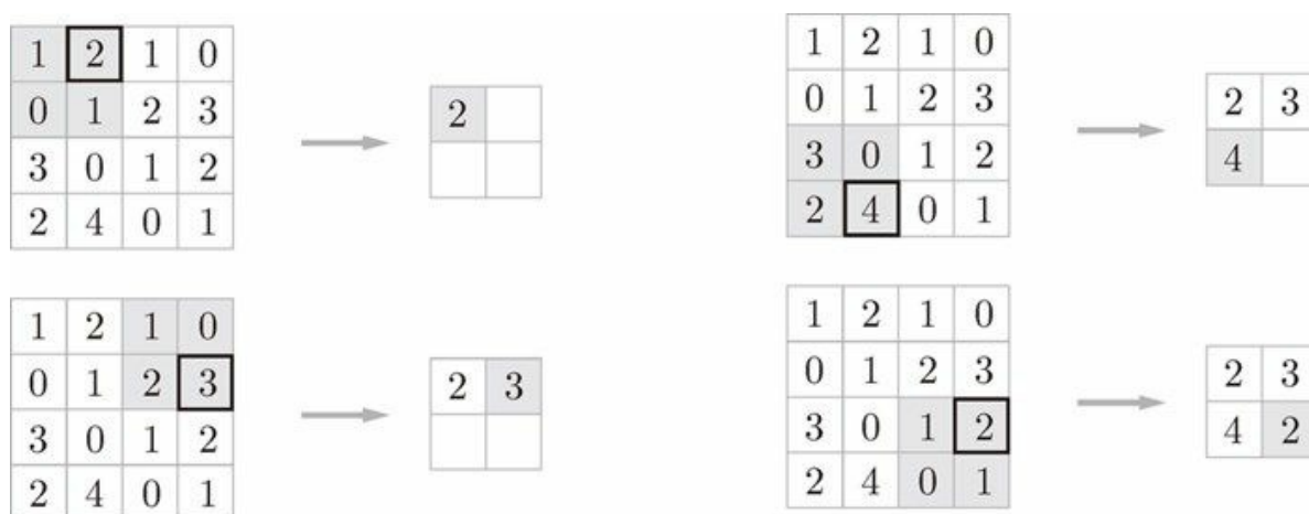
图 7-14 Max 池化的处理顺序
