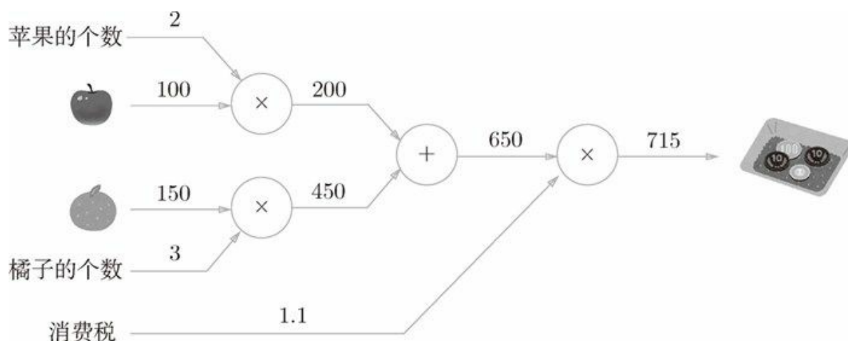
图 5-3 基于计算图求解的问题 2 的答案
