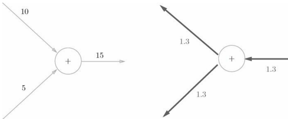
图 5-11 加法节点的反向传播的具体例子
