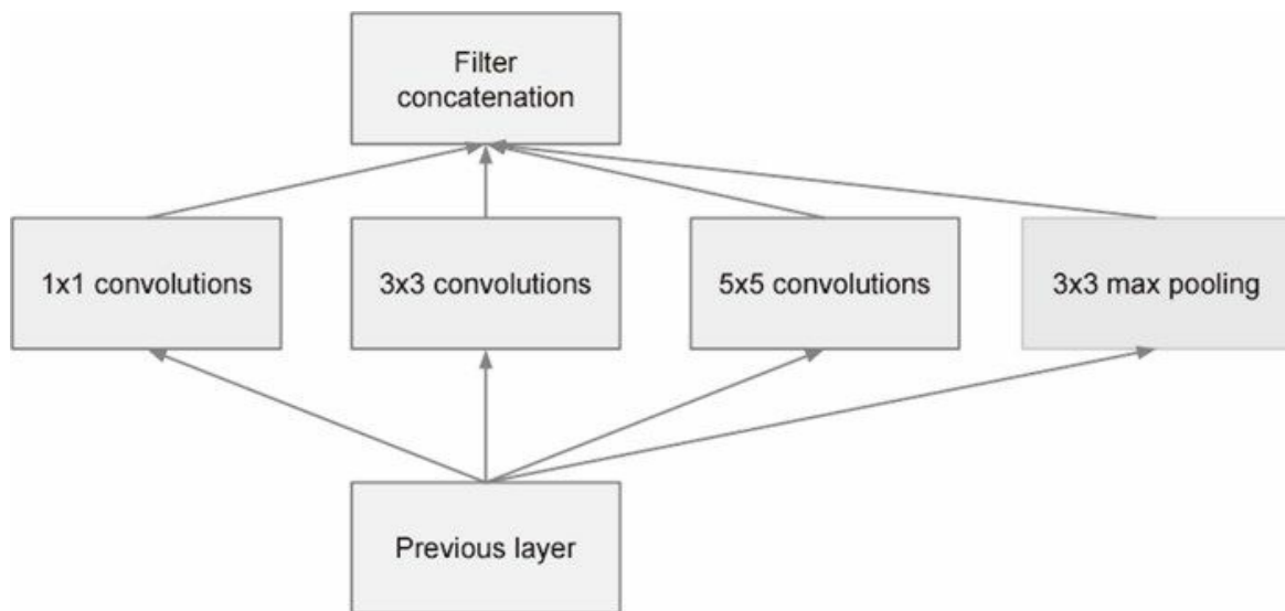
图 8-11 GoogLeNet 的 Inception 结构（引用自文献 [23]）
