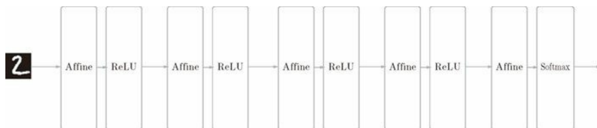
图 7-1 基于全连接层（Affine 层）的网络的例子
