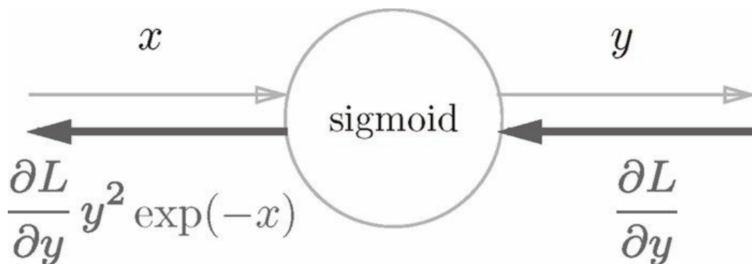
图 5-21 Sigmoid 层的计算图（简洁版）
