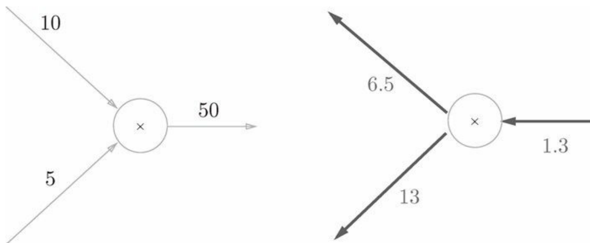
图 5-13 乘法节点的反向传播的具体例子
