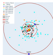
2023년 6월 7일 활동성에 수직 방향으로 배향된 지구 위상점 소행성 위치(아폴로군)
