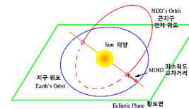
지구 위상점과 지구 근접 거리
