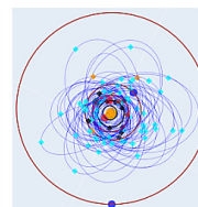
2023년 6월 7일 활동성에 수직 방향으로 배향된 지구 위상점 소행성 위치(아텐군)
