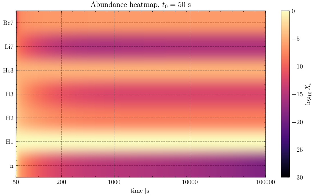
Figura 12: Mapa de abundancias para el modelo t_0 = 50 s.
