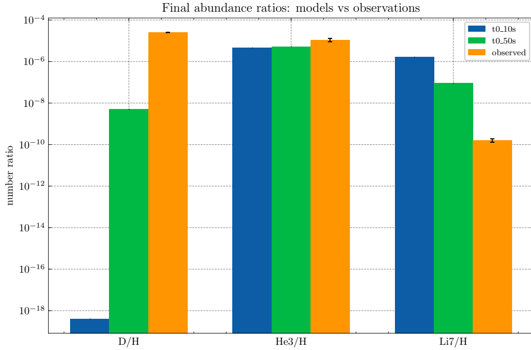
Figura 9: Comparación final de cocientes de abundancia entre los dos modelos y los valores observacionales.
