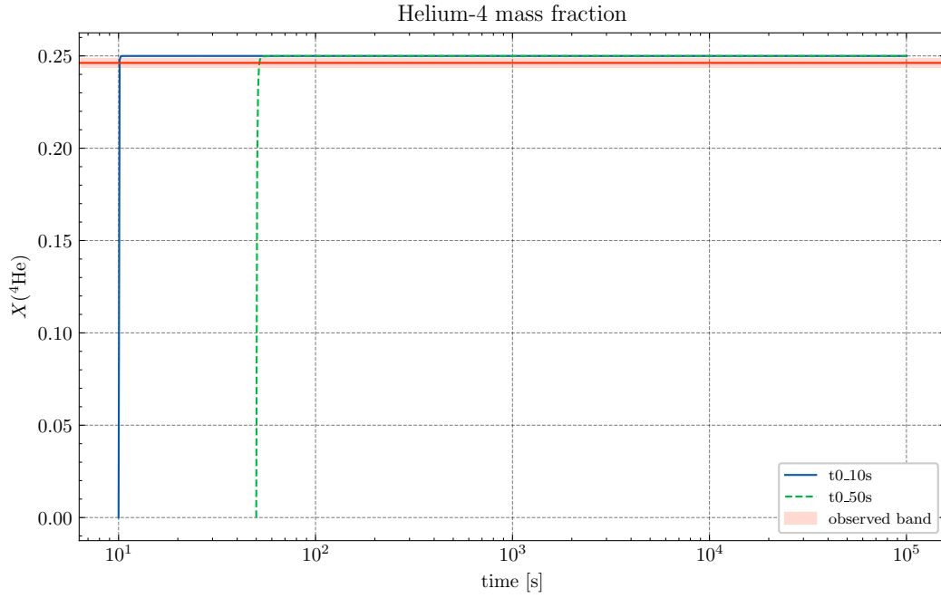
Figura 7: Evolución de la fracción másica X(^4\text{He}) para los dos modelos y comparación con una banda observacional de Y_p .
