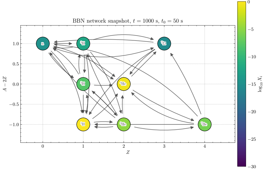
Figura 3: Grafo de red para la simulación t_0 = 50 s evaluado en t = 1000 s.
