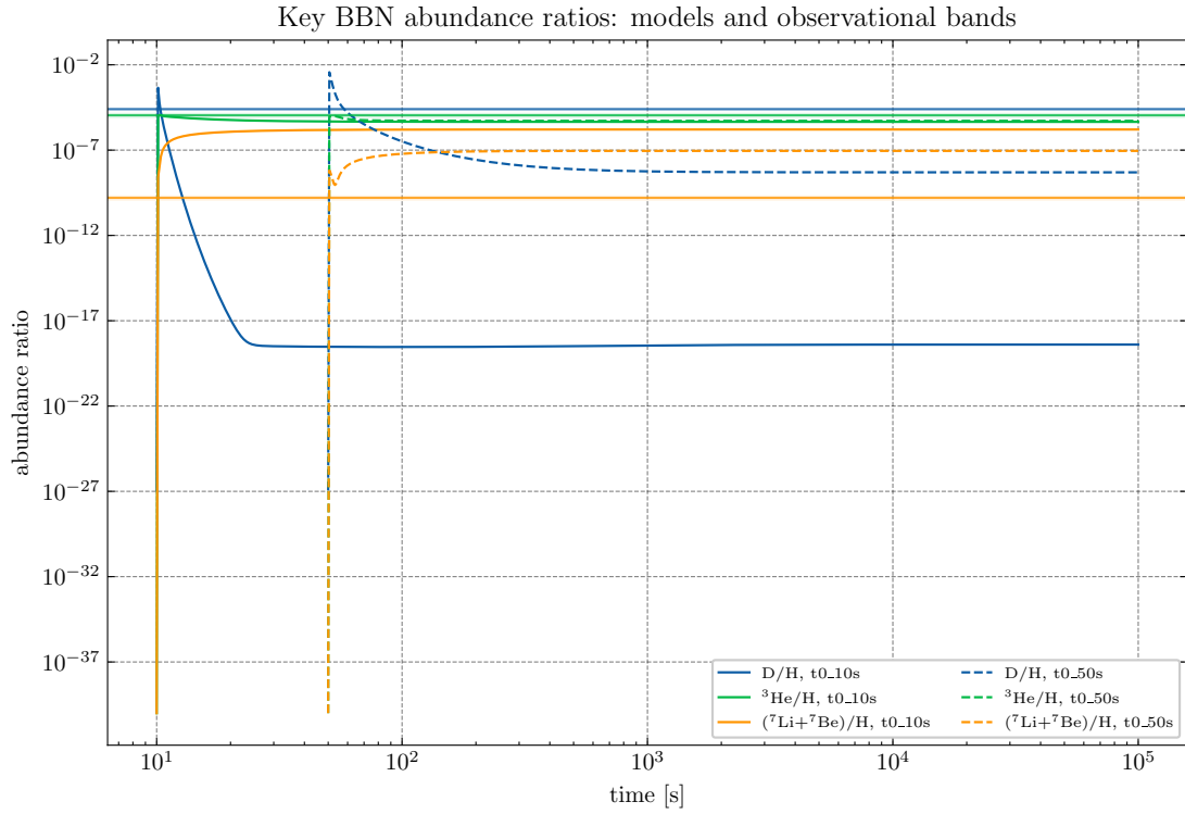
Figura 6: Evolución de D/H , {}^3\text{He}/H y \frac{{}^7\text{Li}+{}^7\text{Be}}{H} para los dos modelos, comparada con las bandas observacionales usadas en el notebook.
