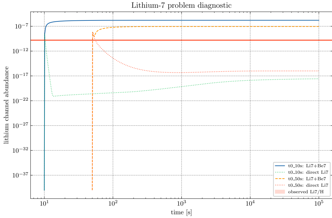
Figura 10: Diagnóstico del canal de masa 7. Se compara la producción de {}^7\text{Li} directo y la suma {}^7\text{Li}+{}^7\text{Be} frente a la banda observacional usada para {}^7\text{Li}/\text{H} .
