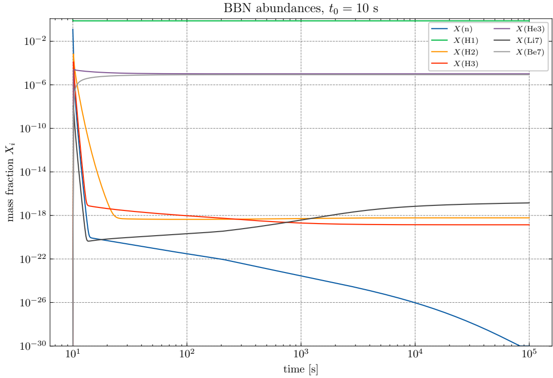
Figura 4: Evolución de todas las fracciones másicas para la simulación iniciada en t_0 = 10 s.
