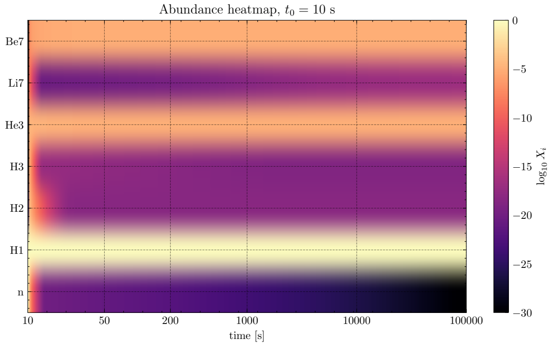
Figura 11: Mapa de abundancias para el modelo t_0 = 10\text{ s} .
