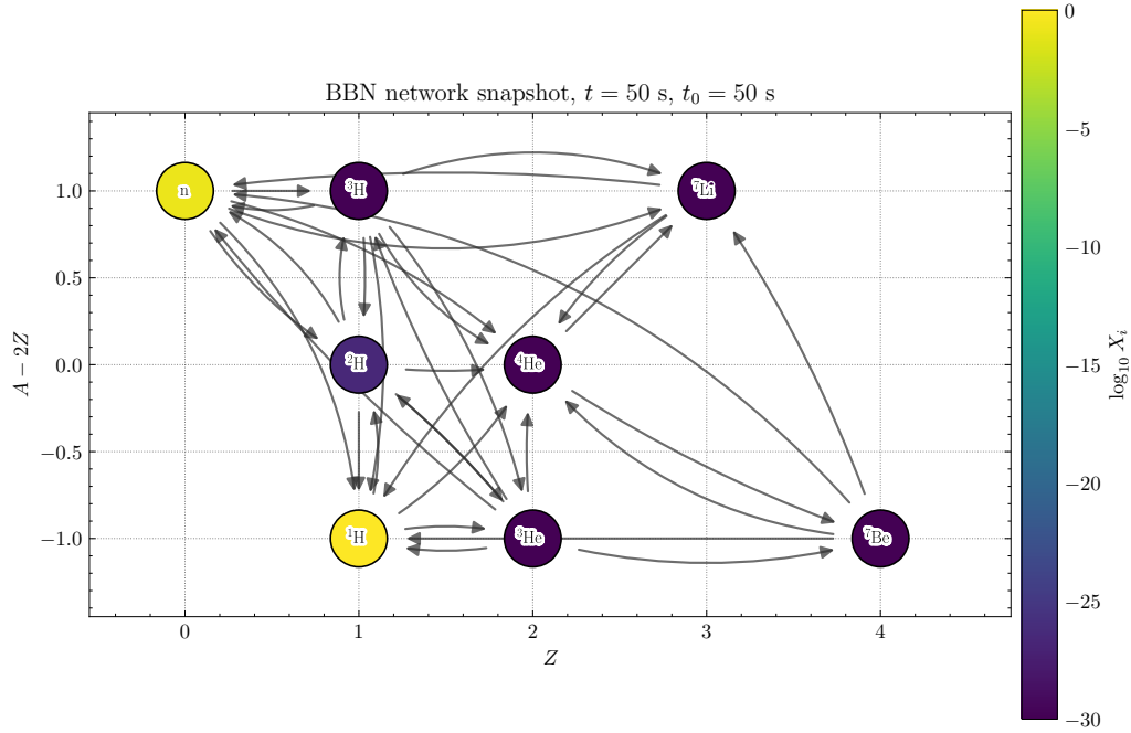
Figura 1: Grafo de red para la simulación t_0 = 50 s evaluado en el primer snapshot, t = 50 s.
