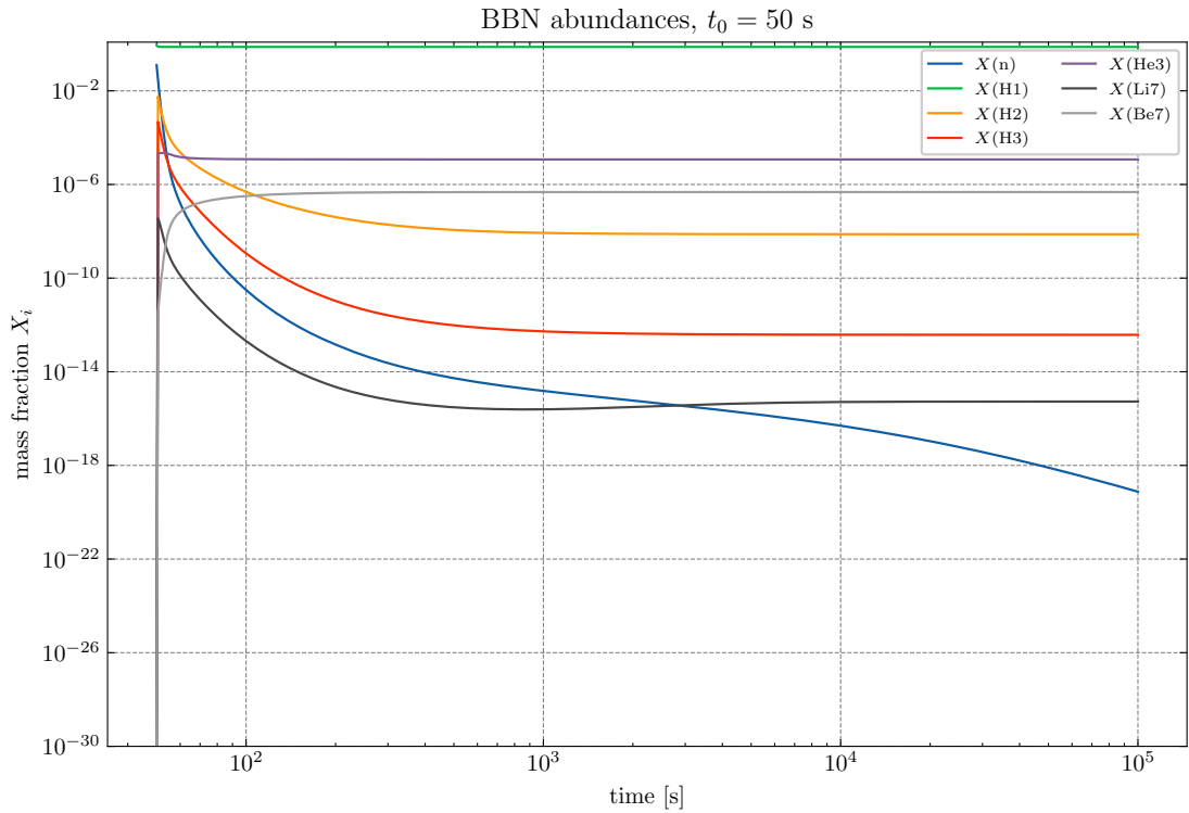
Figura 5: Evolución de todas las fracciones másicas para la simulación iniciada en t_0 = 50 s.
