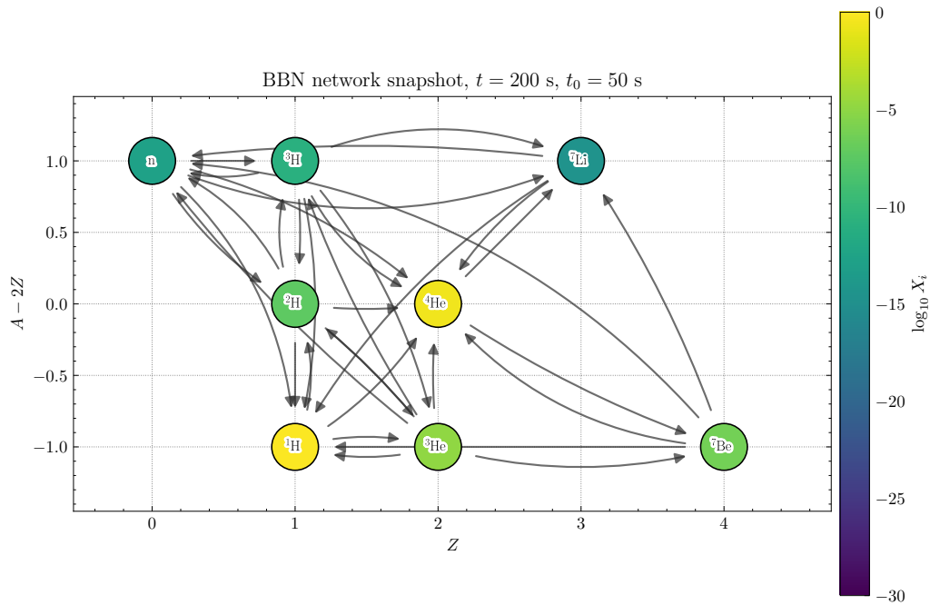
Figura 2: Grafo de red para la simulación t_0 = 50 s evaluado en t = 200 s.
