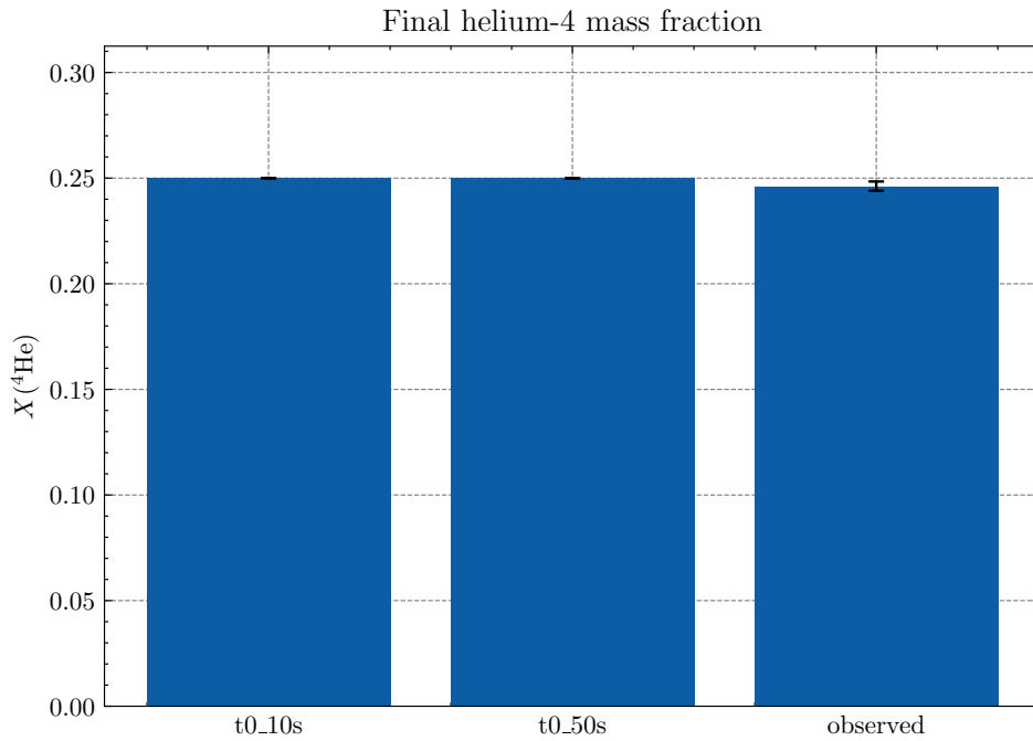
Figura 8: Comparación final de X(^4\text{He}) entre los dos modelos y el valor observacional adoptado.
