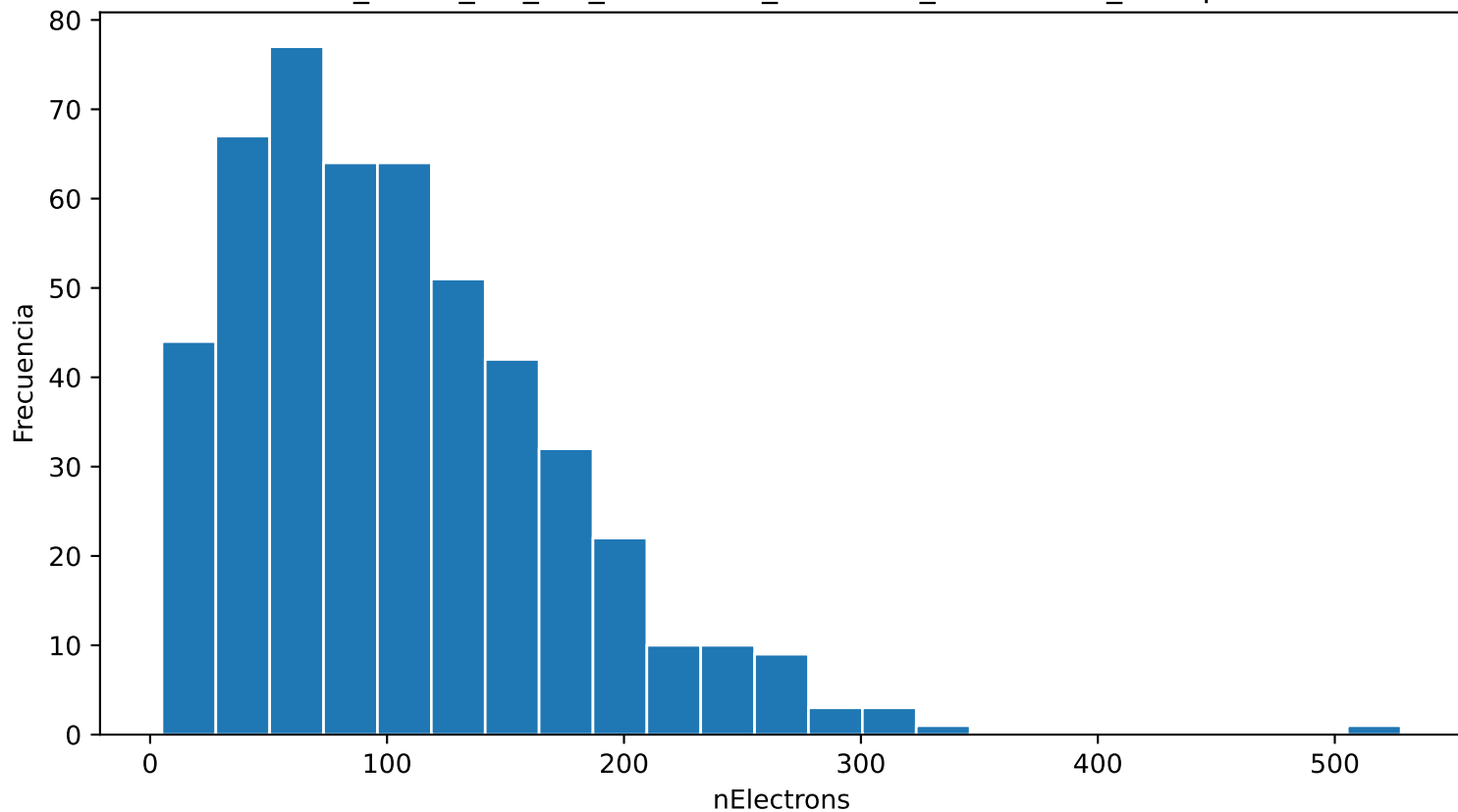
Distribución de nElectrons ar_100.0_cf4_0.0_60.0kVcm_1.000bar_0.0455mm_500npe
