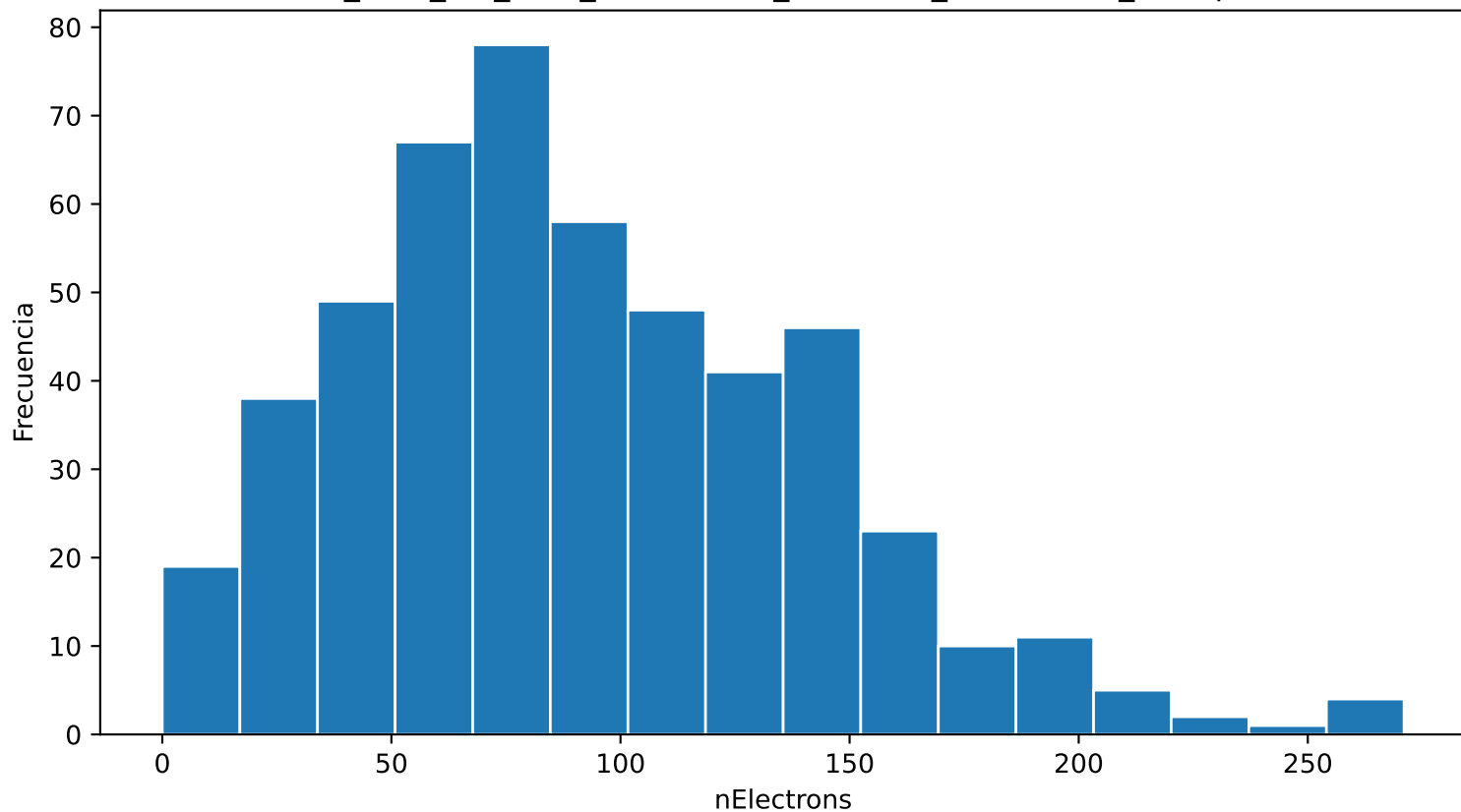
Distribución de nElectrons ar_33.0_cf4_67.0_110.0kVcm_1.000bar_0.0230mm_500npe
