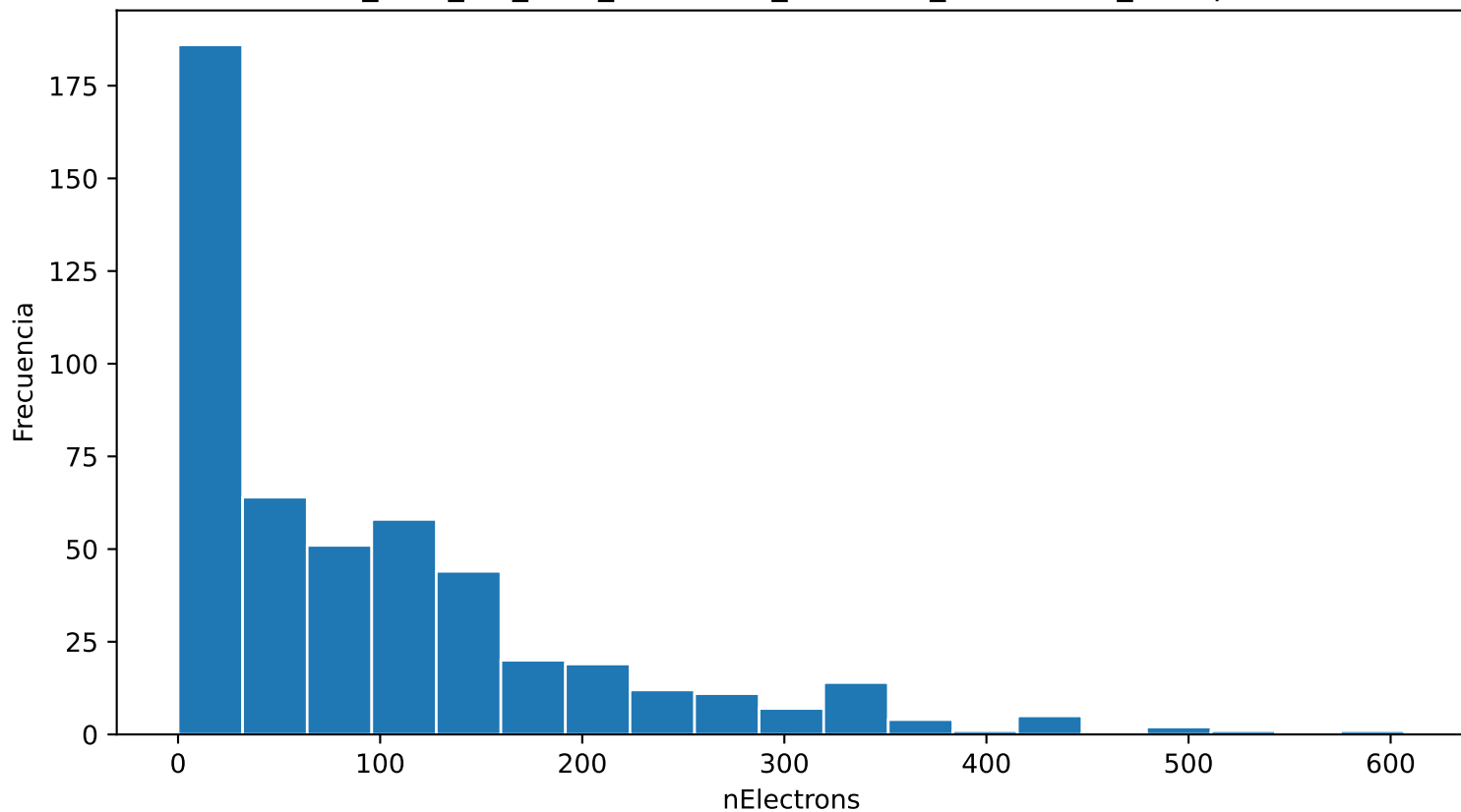
Distribución de nElectrons ar_33.0_cf4_67.0_40.0kVcm_1.000bar_0.2255mm_500npe
