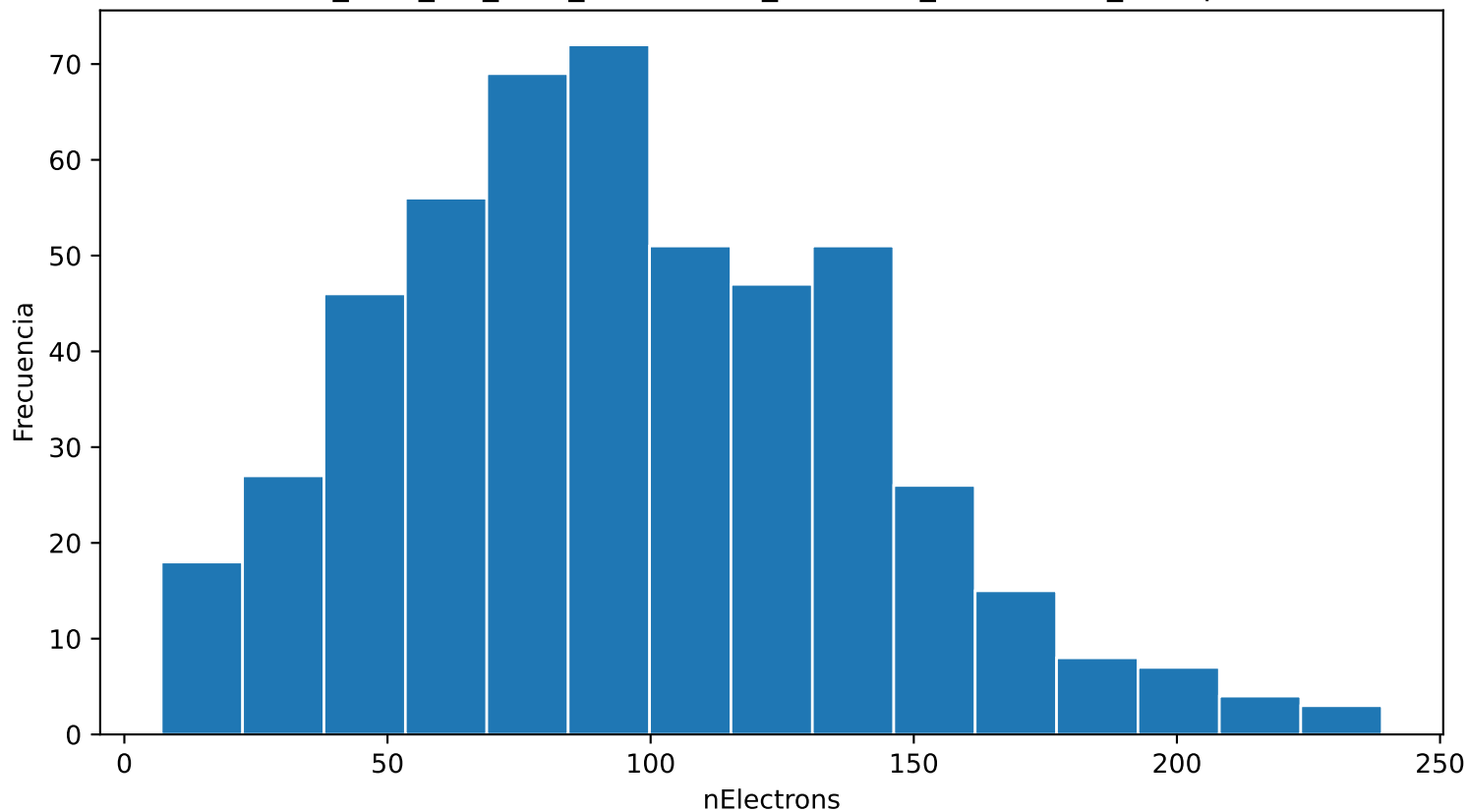
Distribución de nElectrons ar_67.0_cf4_33.0_110.0kVcm_1.000bar_0.0214mm_500npe
