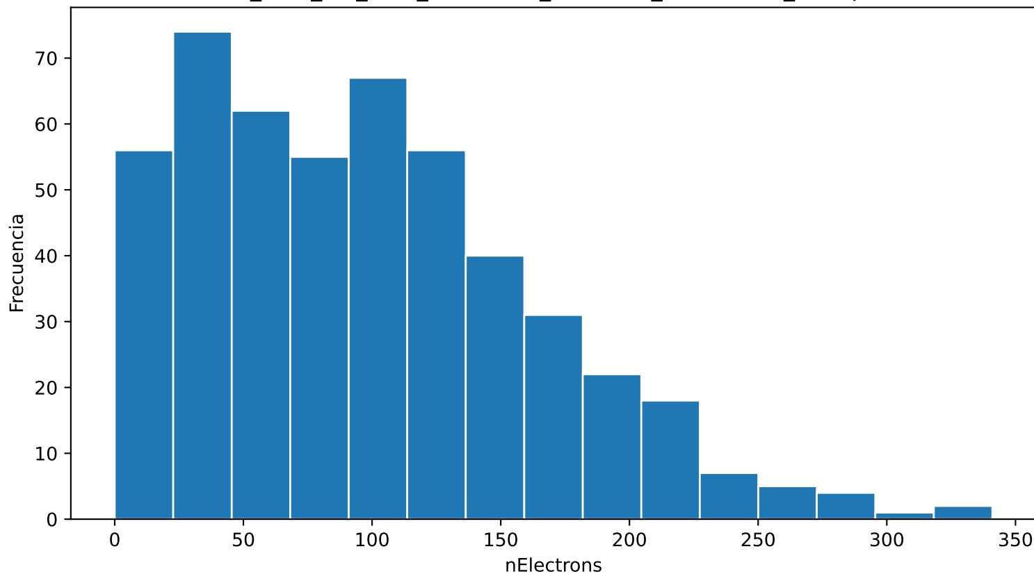
Distribución de nElectrons ar_67.0_cf4_33.0_60.0kVcm_1.000bar_0.0534mm_500npe
