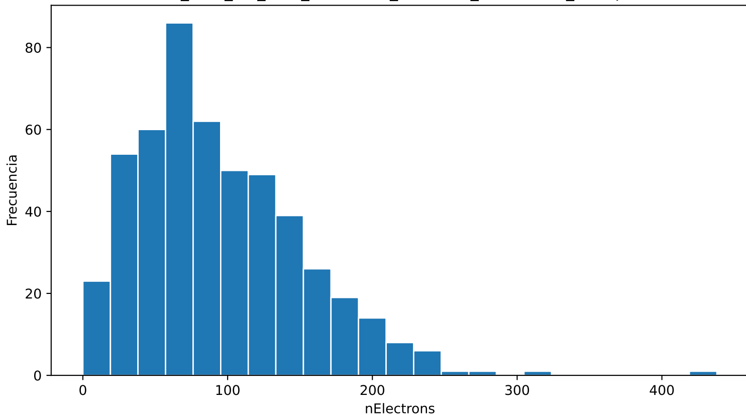
Distribución de nElectrons ar_67.0_cf4_33.0_70.0kVcm_1.000bar_0.0409mm_500npe
