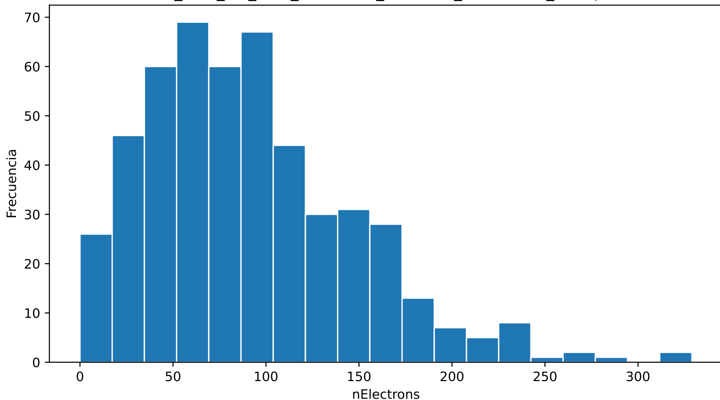
Distribución de nElectrons ar_67.0_cf4_33.0_80.0kVcm_1.000bar_0.0332mm_500npe
