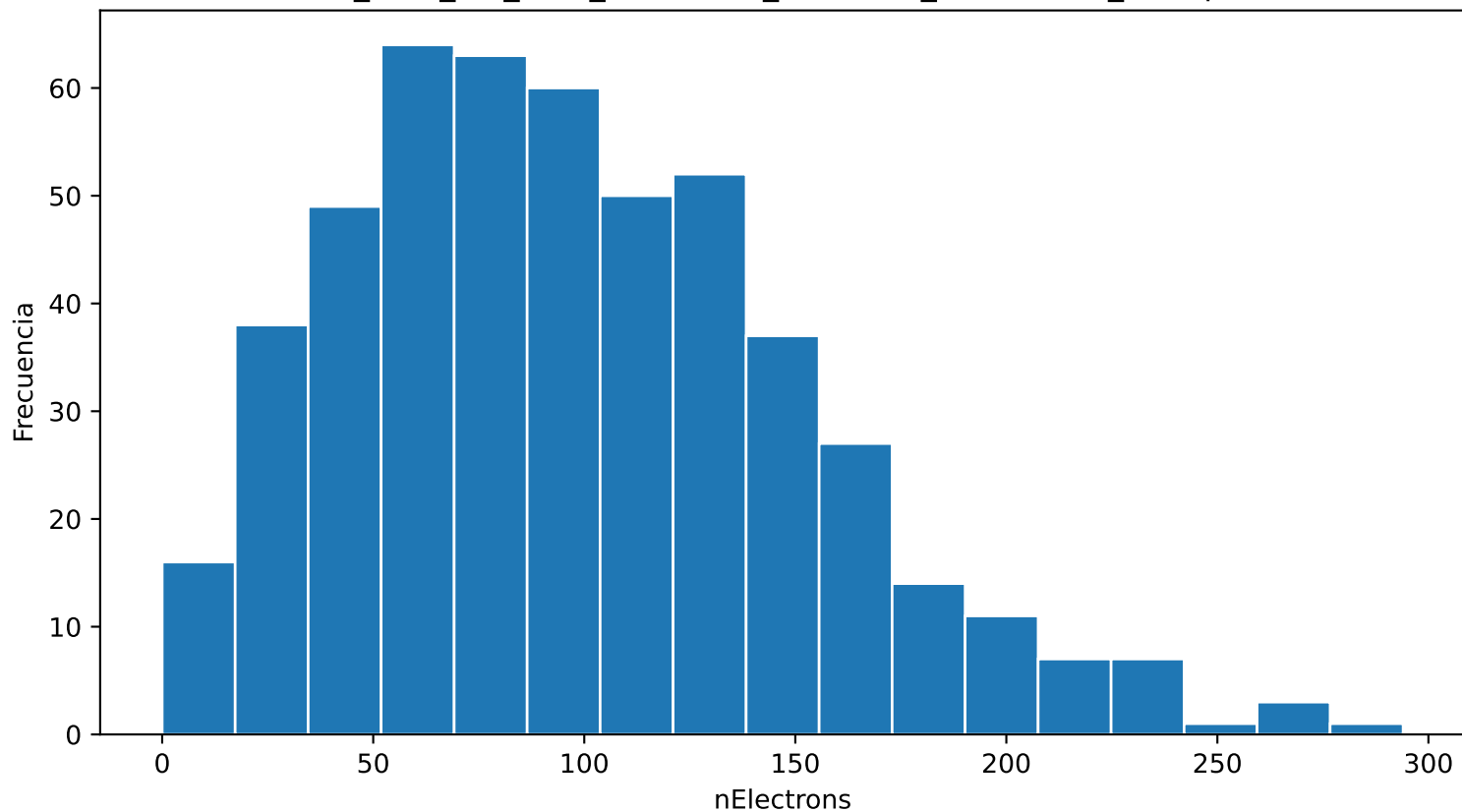
Distribución de nElectrons ar_90.0_cf4_10.0_90.0kVcm_1.000bar_0.0267mm_500npe
