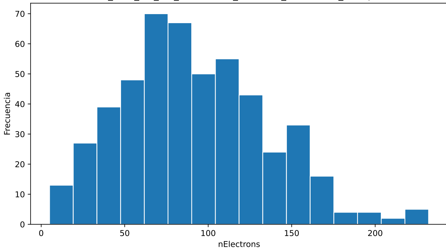
Distribución de nElectrons ar_95.0_cf4_5.0_110.0kVcm_1.000bar_0.0202mm_500npe
