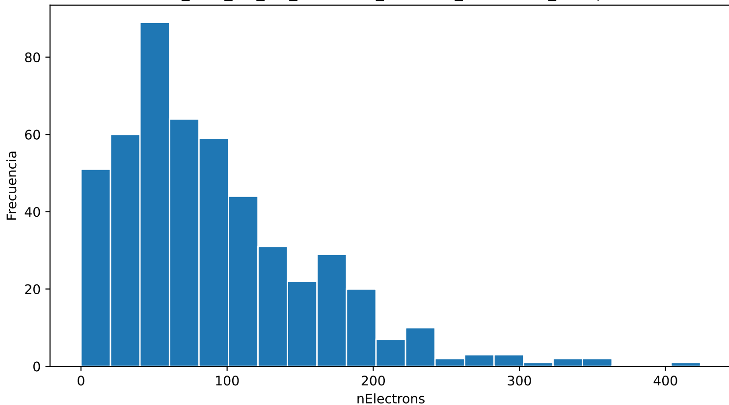
Distribución de nElectrons ar_95.0_cf4_5.0_40.0kVcm_1.000bar_0.0901mm_500npe
