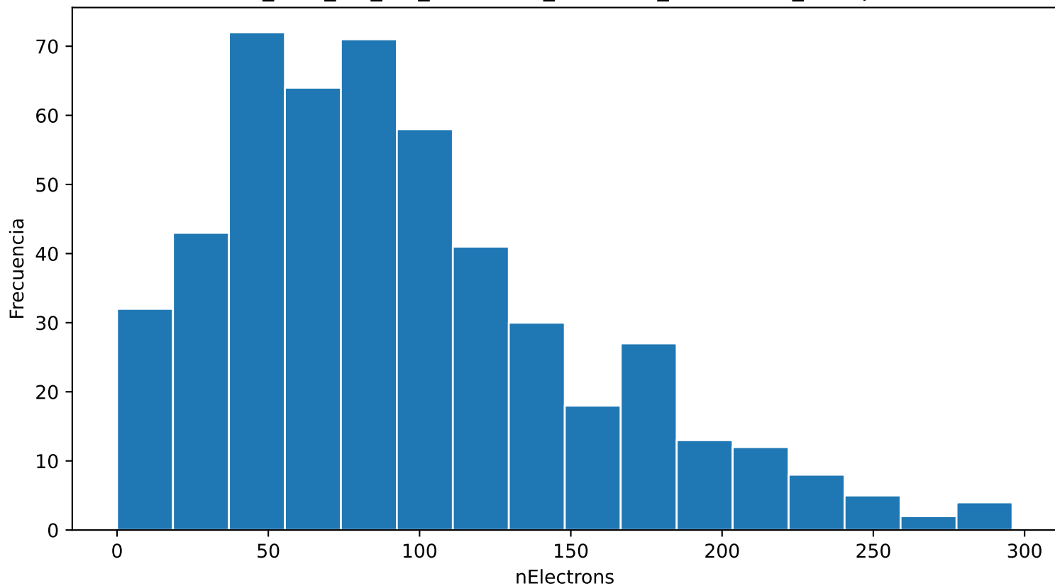
Distribución de nElectrons ar_95.0_cf4_5.0_60.0kVcm_1.000bar_0.0461mm_500npe
