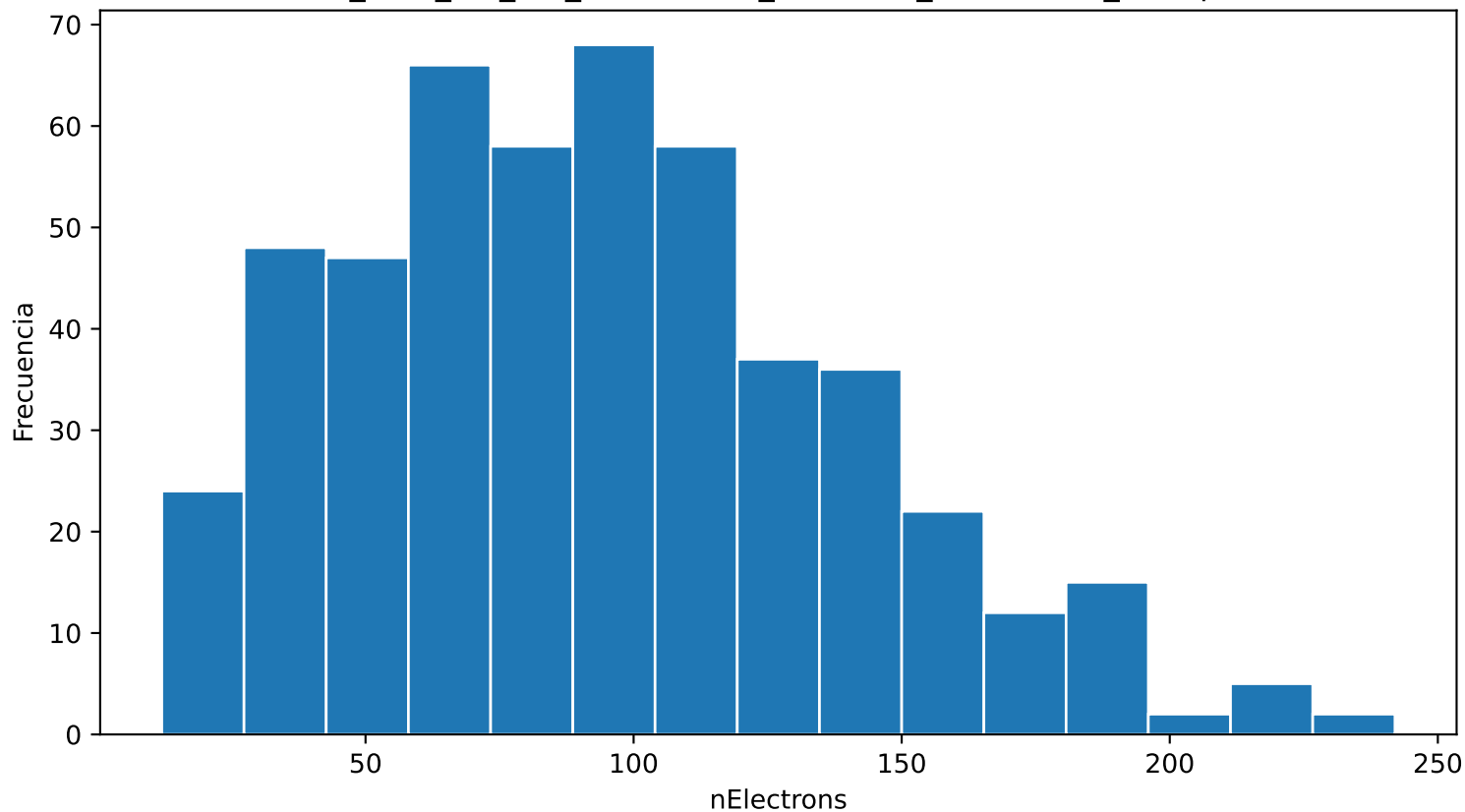
Distribución de nElectrons ar_99.0_cf4_1.0_110.0kVcm_1.000bar_0.0201mm_500npe
