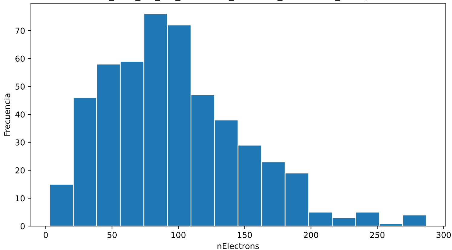
Distribución de nElectrons ar_99.0_cf4_1.0_90.0kVcm_1.000bar_0.0259mm_500npe
