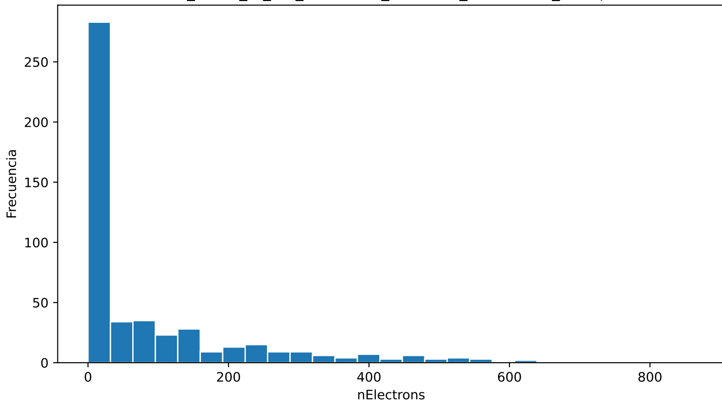
Distribución de nElectrons cf4_100.0_ar_0.0_40.0kVcm_1.000bar_0.5086mm_500npe
