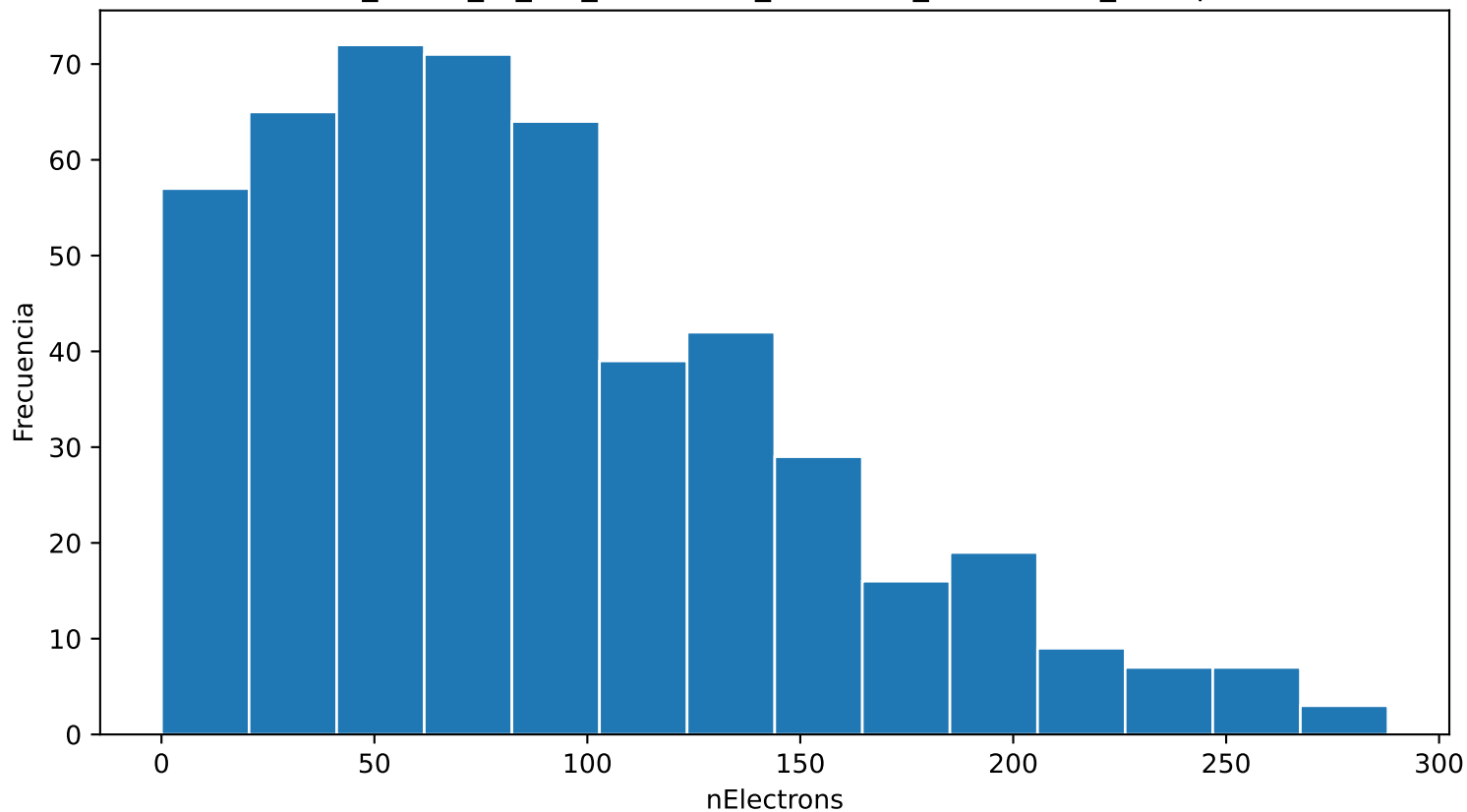
Distribución de nElectrons cf4_100.0_ar_0.0_80.0kVcm_1.000bar_0.0428mm_500npe
