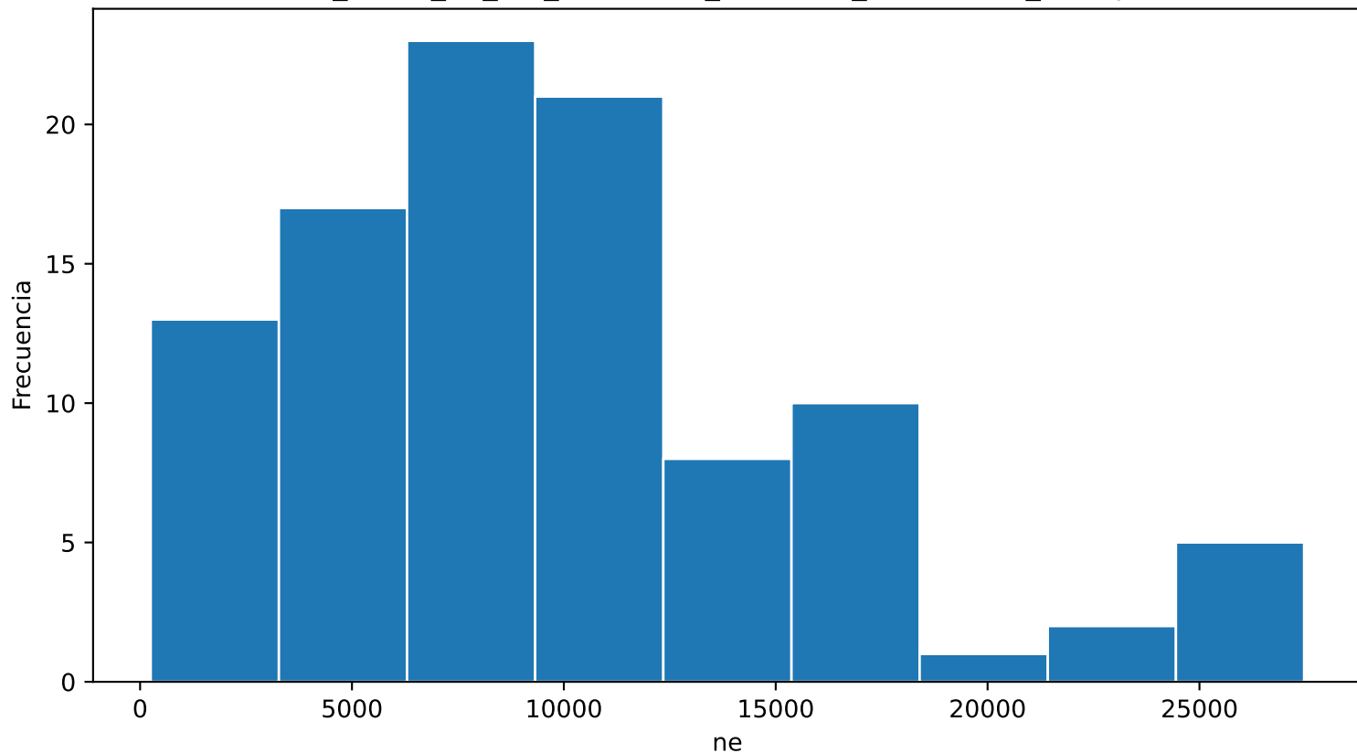
Distribución de ne ar_100.0_n2_0.0_70.0kVcm_1.000bar_0.0722mm_100npe
