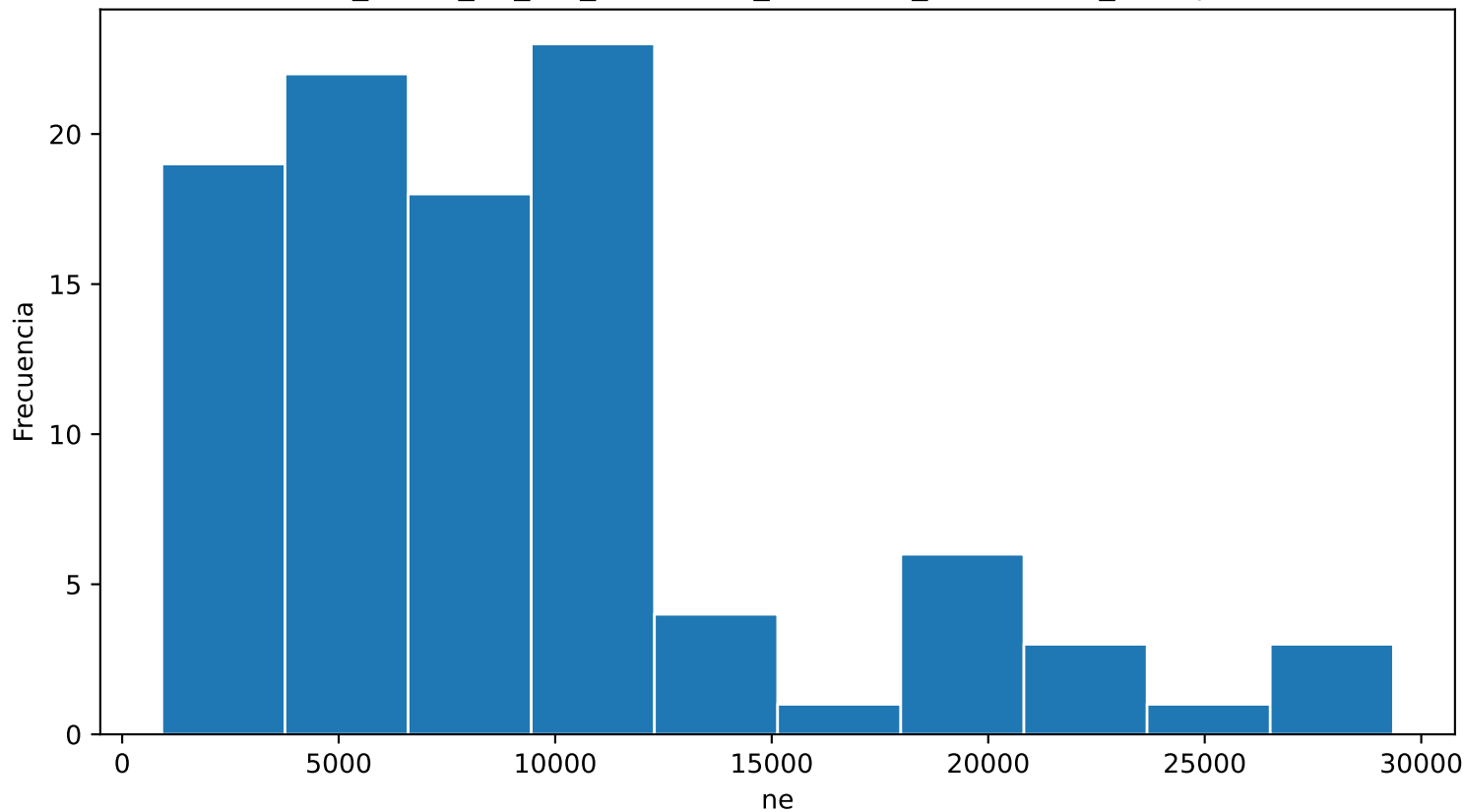
Distribución de ne ar_100.0_n2_0.0_90.0kVcm_1.000bar_0.0516mm_100npe
