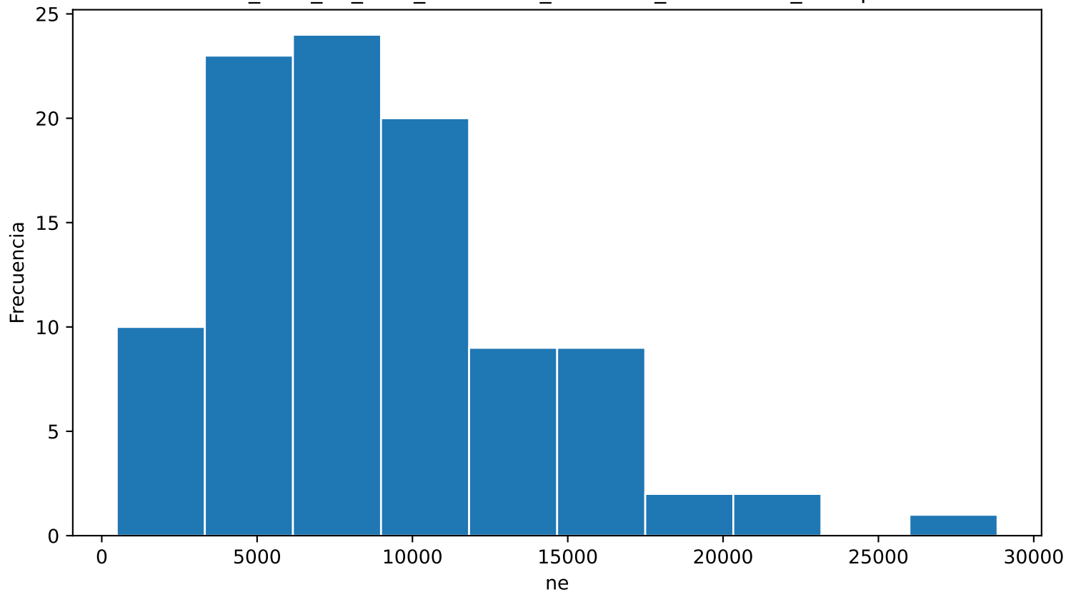
Distribución de ne ar_90.0_n2_10.0_70.0kVcm_1.000bar_0.0832mm_100npe
