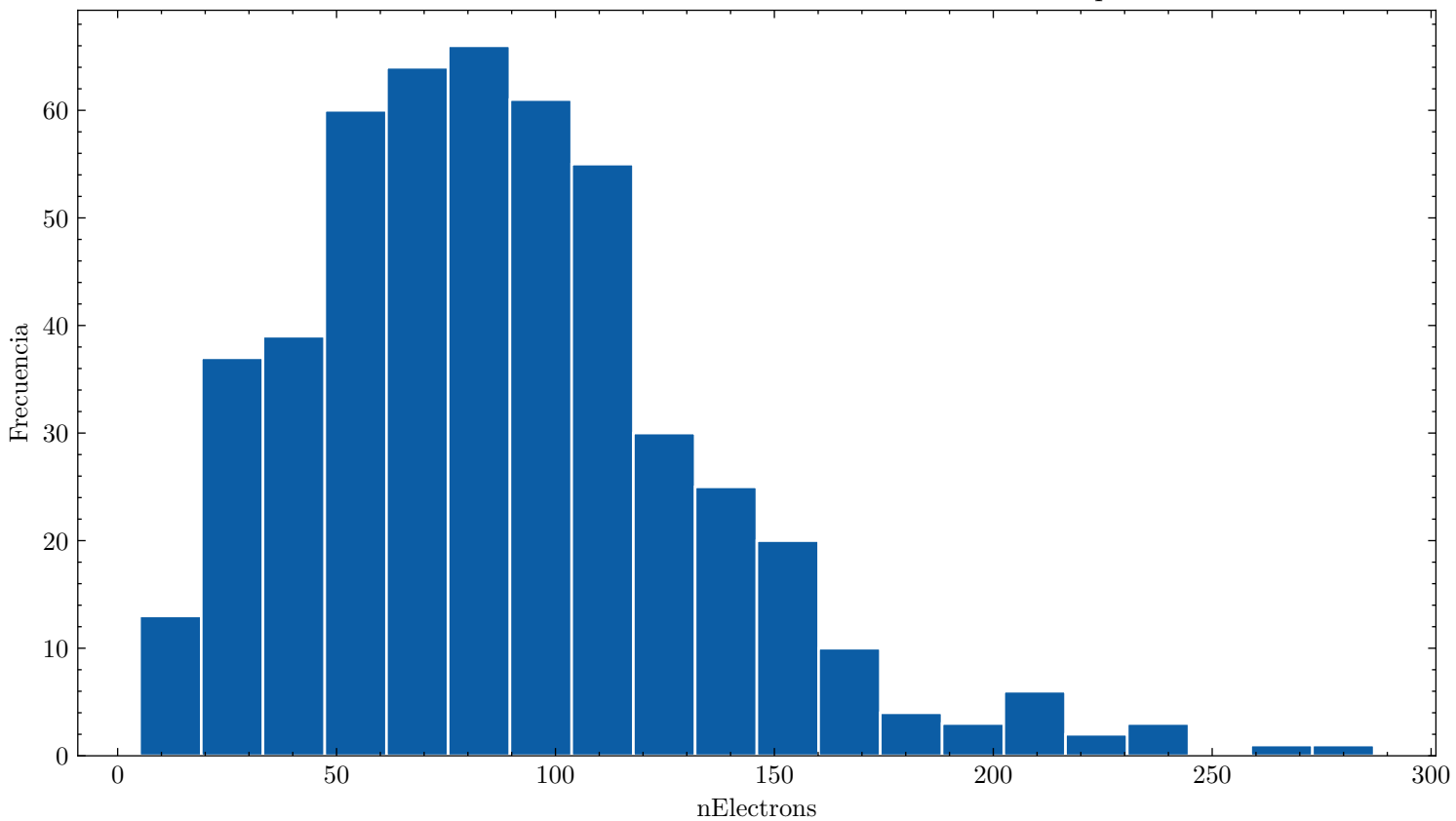
Distribución de nElectrons ar_100.0_cf4_0.0_110.0kVcm_1.000bar_0.0199mm_500npe
