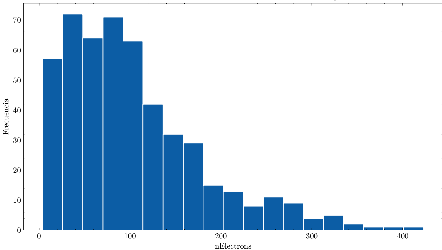
Distribución de nElectrons ar_100.0_cf4_0.0_40.0kVcm_1.000bar_0.0871mm_500npe
