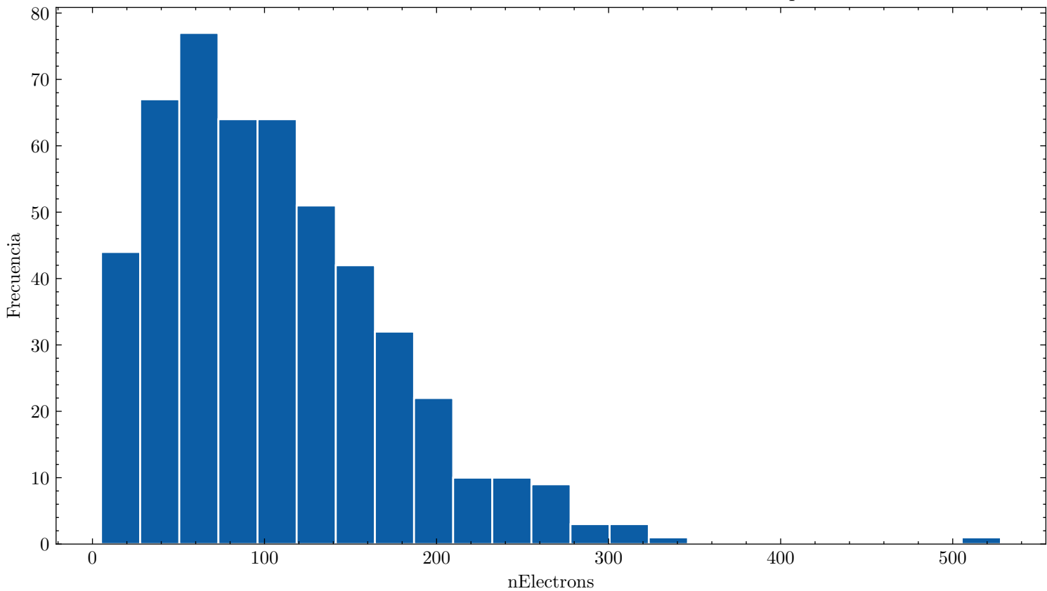
Distribución de nElectrons ar_100.0_cf4_0.0_60.0kVcm_1.000bar_0.0455mm_500npe
