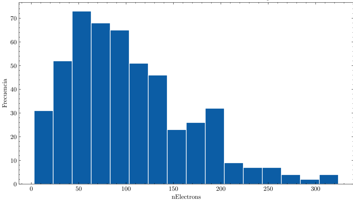
Distribución de nElectrons ar_100.0_cf4_0.0_70.0kVcm_1.000bar_0.0364mm_500npe
