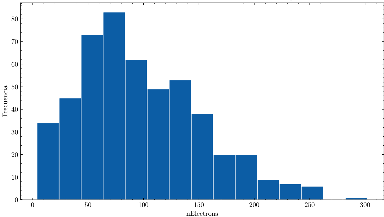
Distribución de nElectrons ar_100.0_cf4_0.0_80.0kVcm_1.000bar_0.0302mm_500npe
