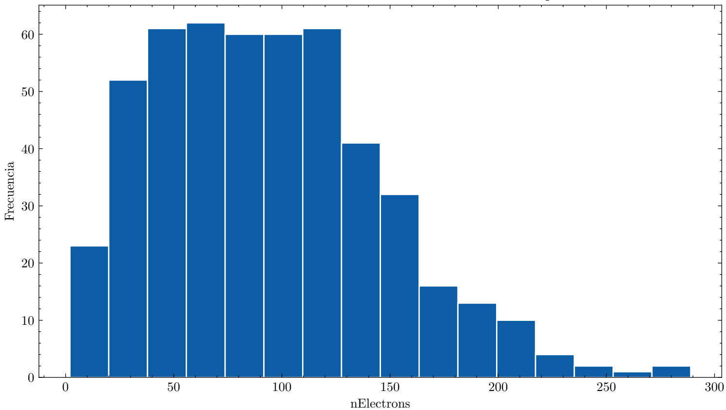
Distribución de nElectrons ar_100.0_cf4_0.0_90.0kVcm_1.000bar_0.0258mm_500npe
