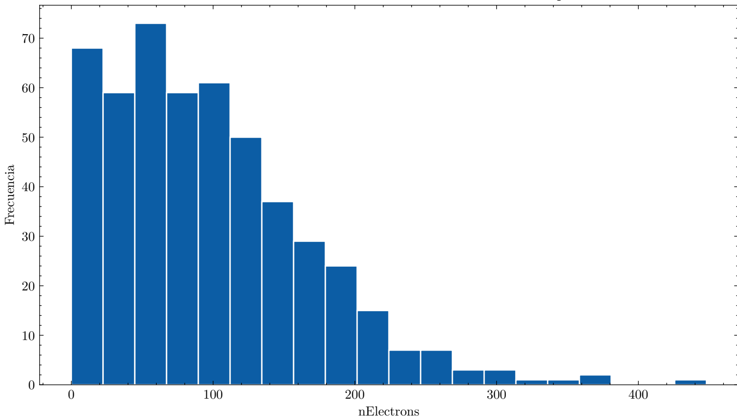
Distribución de nElectrons ar_33.0_cf4_67.0_60.0kVcm_1.000bar_0.0653mm_500npe
